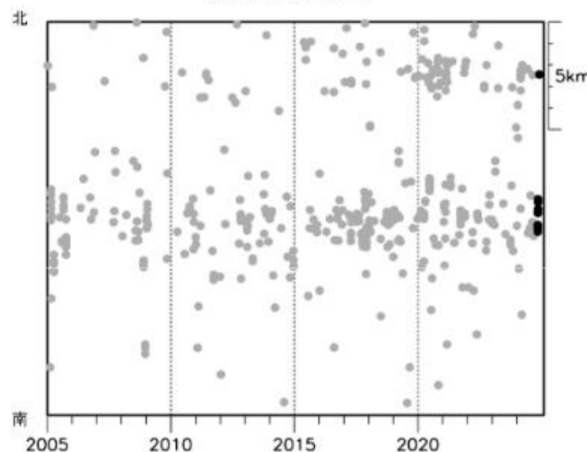
時空間分布図
