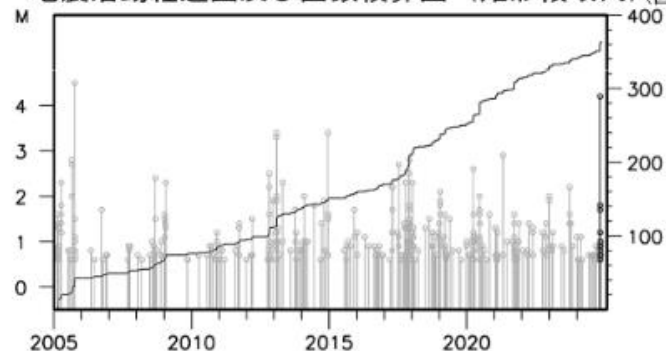
地震活動経過図及び回数積算図（矩形領域内）(回)
