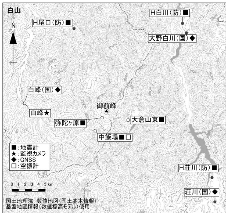
図3 白山観測点配置図
