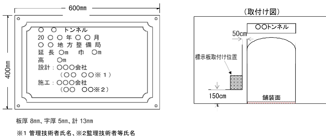
図 6-7-2 標示板の設置イメージ図
