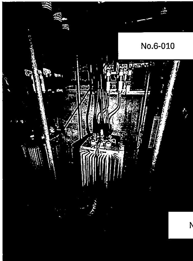
単相変圧器 100kVA×2 全体図
