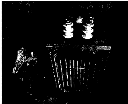
トランス及びコンデンサーの保管状況 屋外物置内
