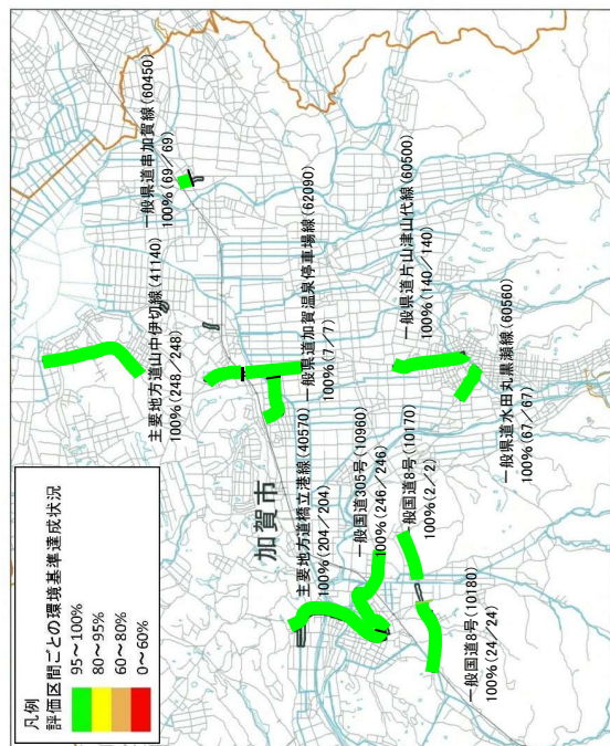
図4-17 センサス区間ごとの環境基準達成状況 加賀市屋間
