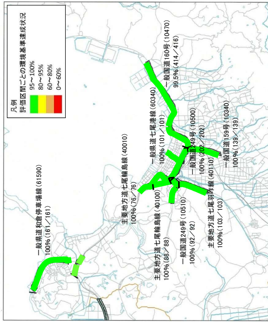
図4-3 センサス区間ごとの環境基準達成状況 七尾市 (旧七尾市) 昼間
