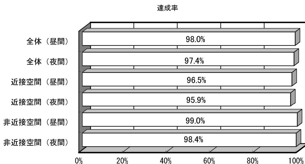
図2-4 時間帯別の達成状況
