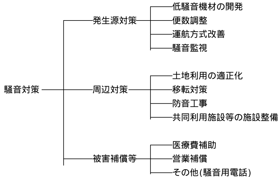
図 - 1 航空機騒音対策の概要
