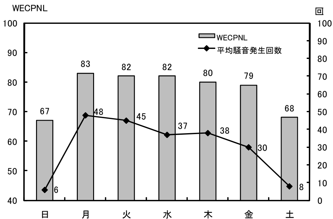
図-7 常時測定点における曜日別1日平均騒音発生回数とWECPNL (No.1 小松市小島町)
