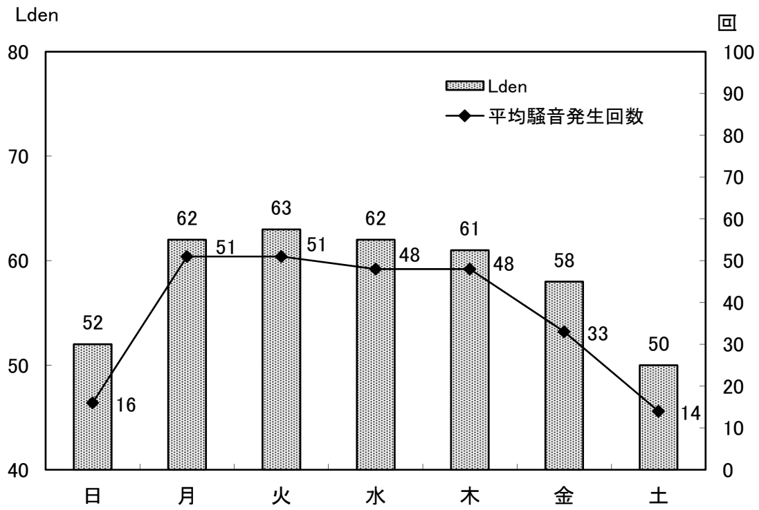
図-8 常時測定点における曜日別1日平均騒音発生回数とLden (No.2 加賀市伊切町)
