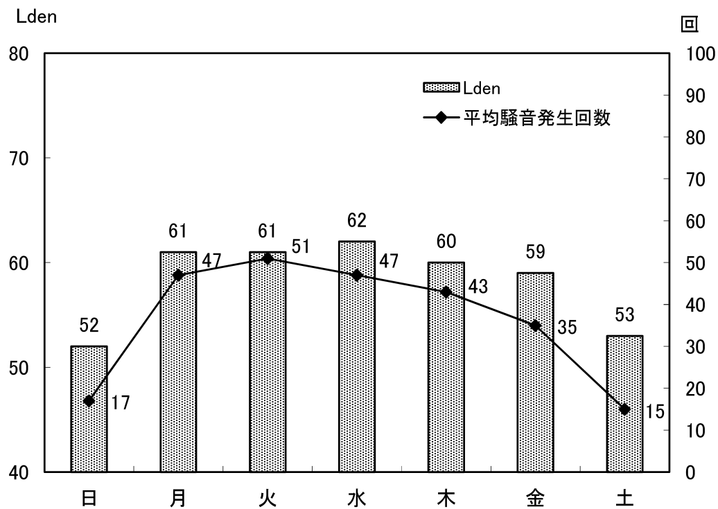
図-8 常時測定点における曜日別1日平均騒音発生回数とLden (No.2 加賀市伊切町)
