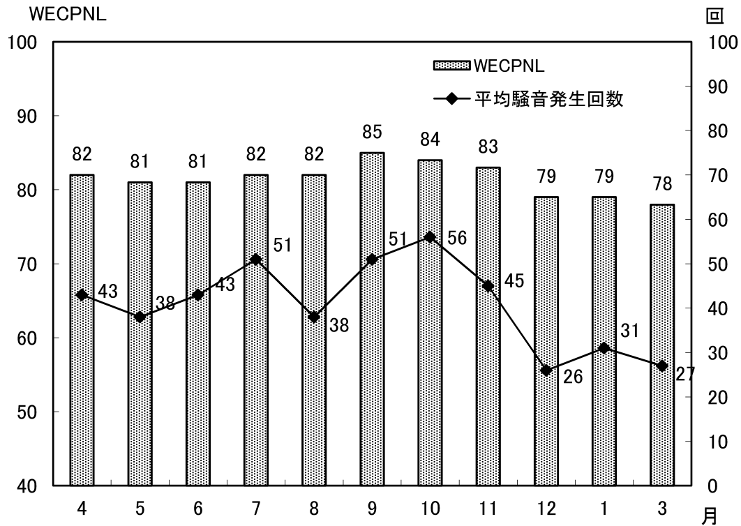
図-10 常時測定点における月別1日平均騒音発生回数とWECPNL (No. 1 小松市小島町)
