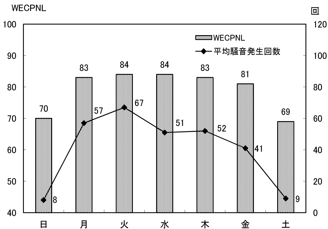
図-12 常時測定点における曜日別1日平均騒音発生回数とWECPNL (No. 1 小松市小島町)
