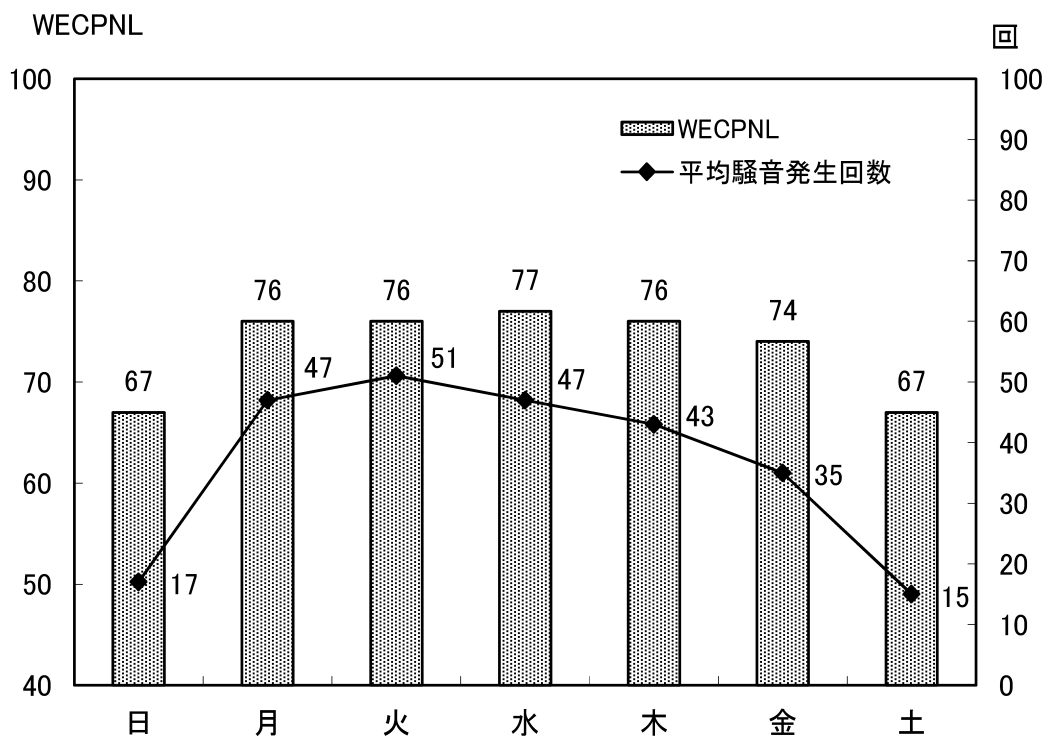
図-13 常時測定点における曜日別1日平均騒音発生回数とWECPNL (No. 2 加賀市伊切町)
