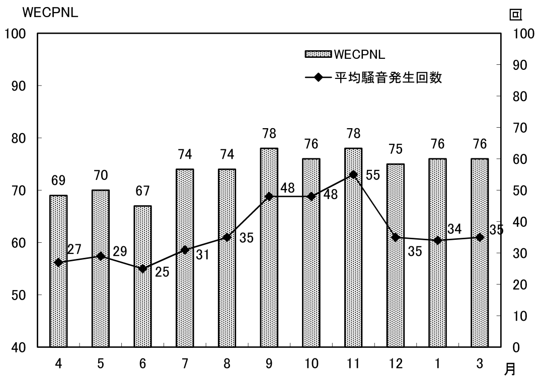
図-11 常時測定点における月別1日平均騒音発生回数とWECPNL (No. 2 加賀市伊切町)
