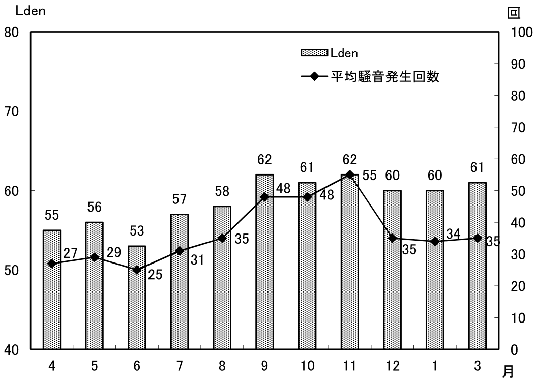
図-6 常時測定点における月別1日平均騒音発生回数とLden (No.2 加賀市伊切町)
