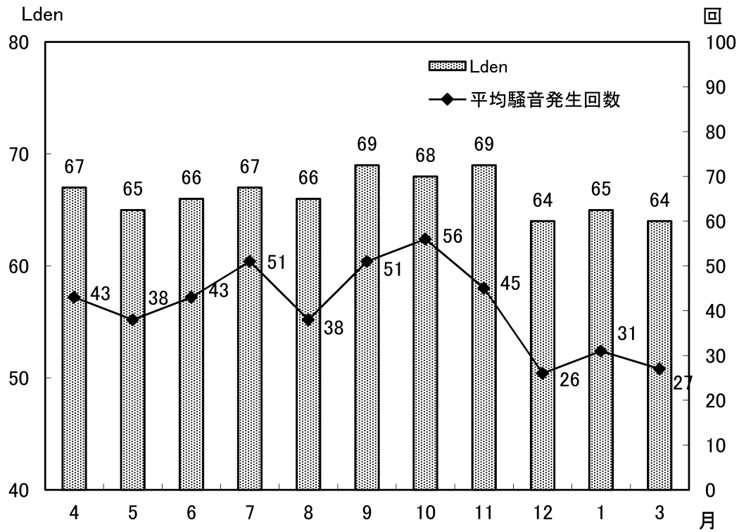
図-5 常時測定点における月別1日平均騒音発生回数とLden (No.1 小松市小島町)
