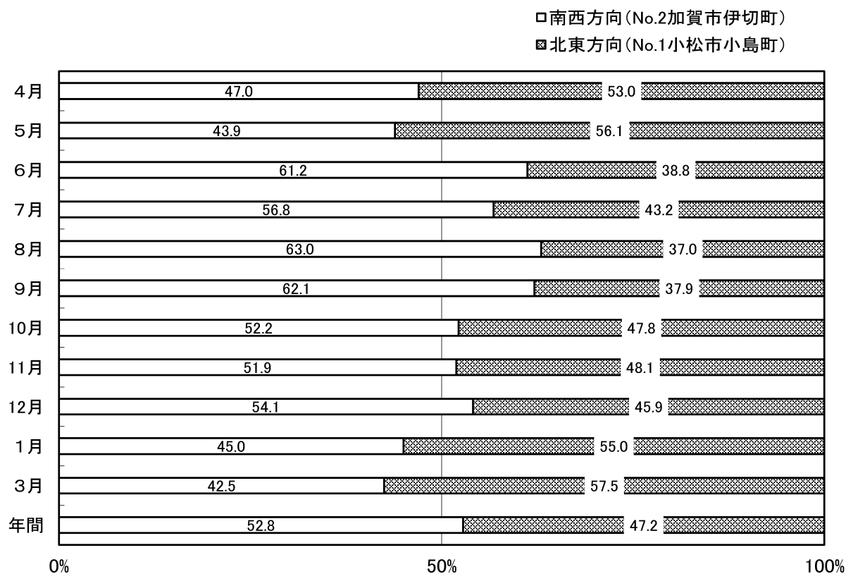
図-3 常時測定点における方向別騒音発生割合
