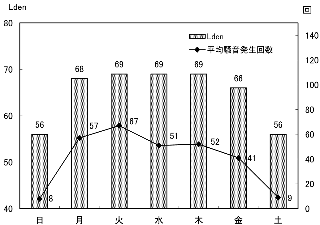
図-7 常時測定点における曜日別1日平均騒音発生回数とLden (No.1 小松市小島町)
