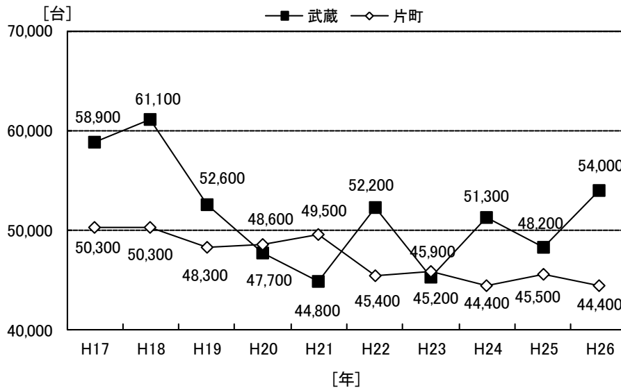
図1-12 金沢市内主要交差点の全方向流入交通量推移
