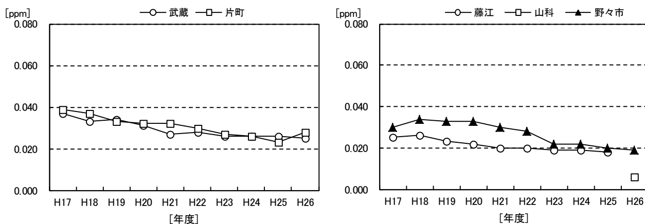
図1-13 二酸化窒素年平均値の経年変化
