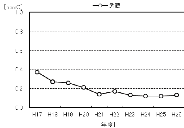
図 1-17 非メタン炭化水素の午前 6 時から 9 時における年平均値の経年変化
