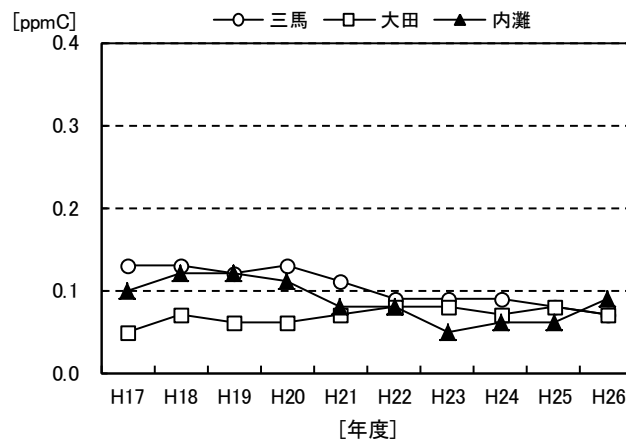
図 1-11 非メタン炭化水素の午前 6 時から 9 時における年平均値の経年変化
