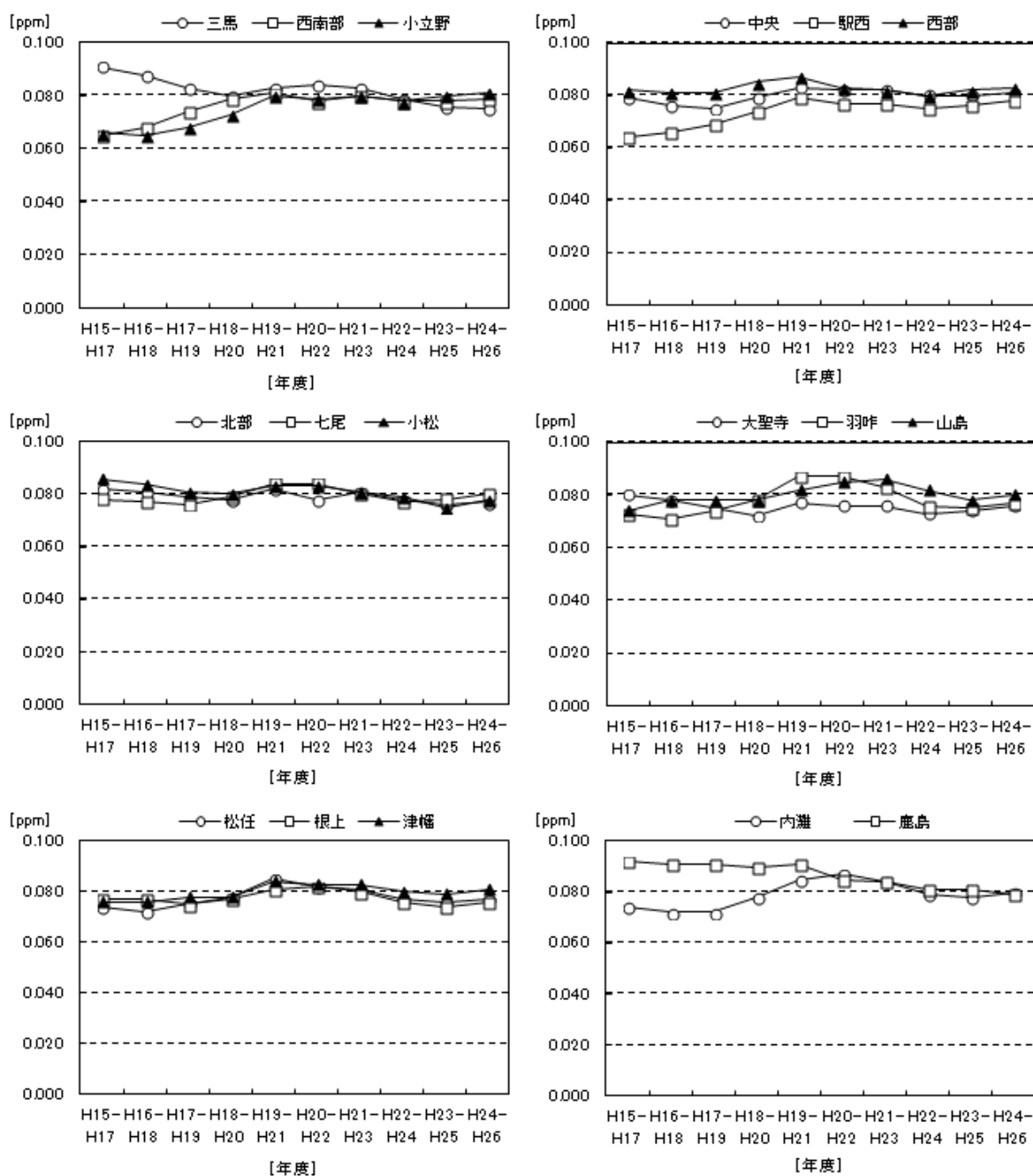
図 1-8 光化学オキシダント濃度 8 時間値の日最高値の年間 99 パーセンタイル値の 3 年平均値
