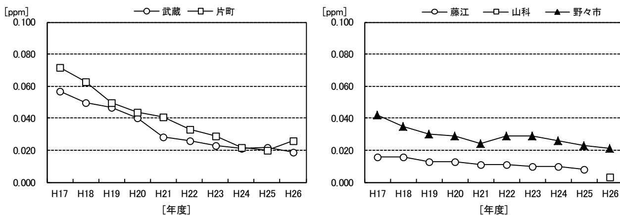
図 1-14 一酸化窒素年平均値の経年変化
