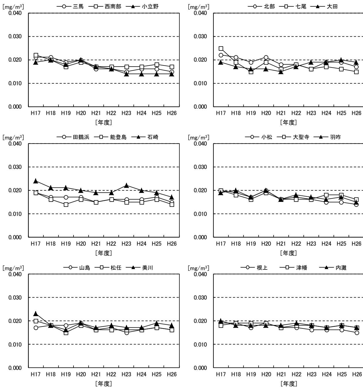
図1-9 10年間継続測定局における浮遊粒子状物質年平均値の経年変化
