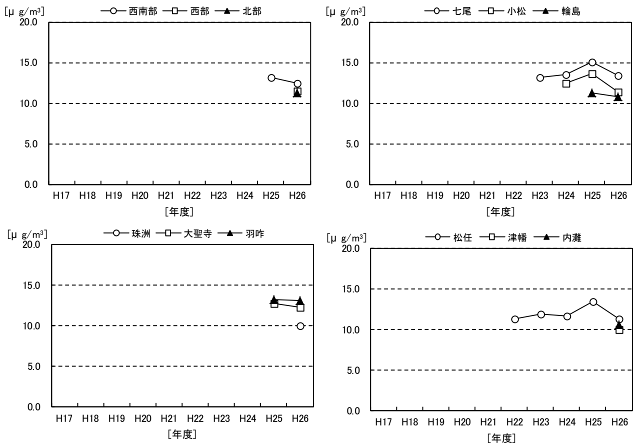
図 1-10 微小粒子状物質年平均値の経年変化
