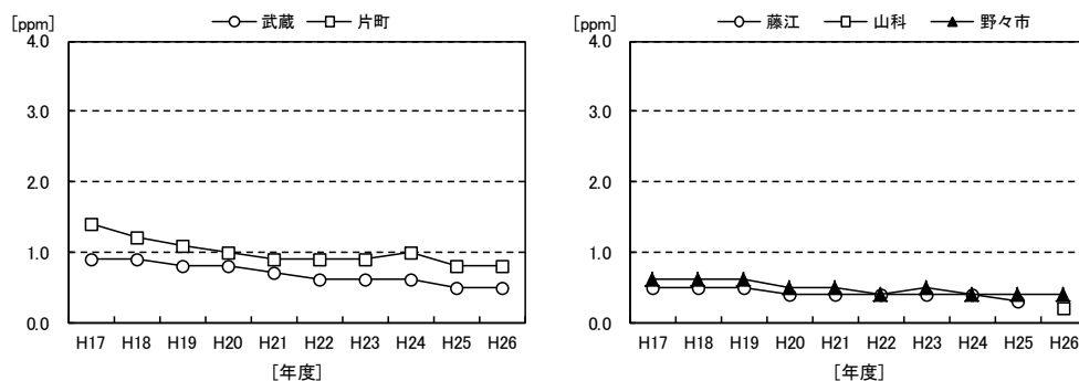
図 1-15 一酸化炭素年平均値の経年変化
