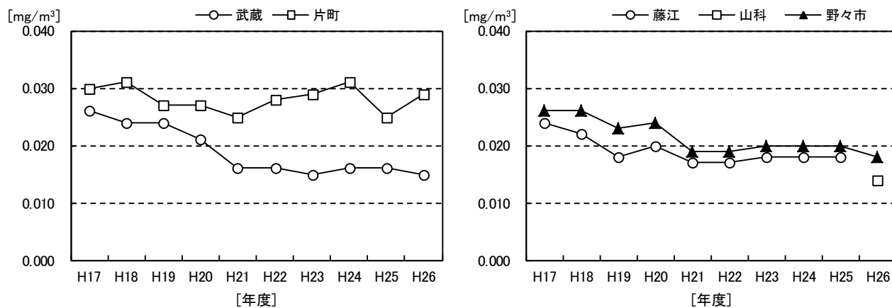
図1-16 浮遊粒子状物質年平均値の経年変化
