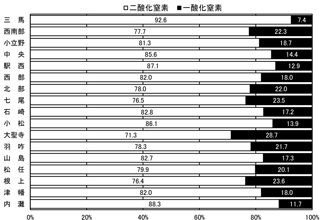
図 1-5 一般環境大気測定局における二酸化窒素と一酸化窒素の比率(平成 26 年度)
