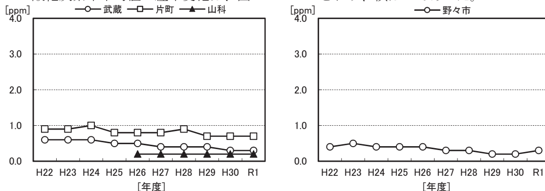
図 1-16 一酸化炭素年平均値の経年変化
