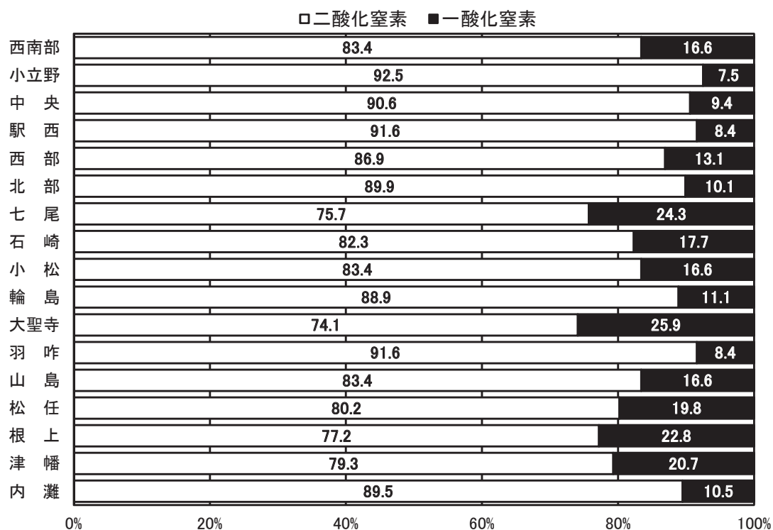
図 1-5 一般環境大気測定局における二酸化窒素と一酸化窒素の比率(令和元年度)
