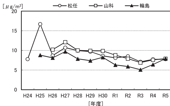
図 3－1 PM2.5 の質量濃度年平均値の経年変化
