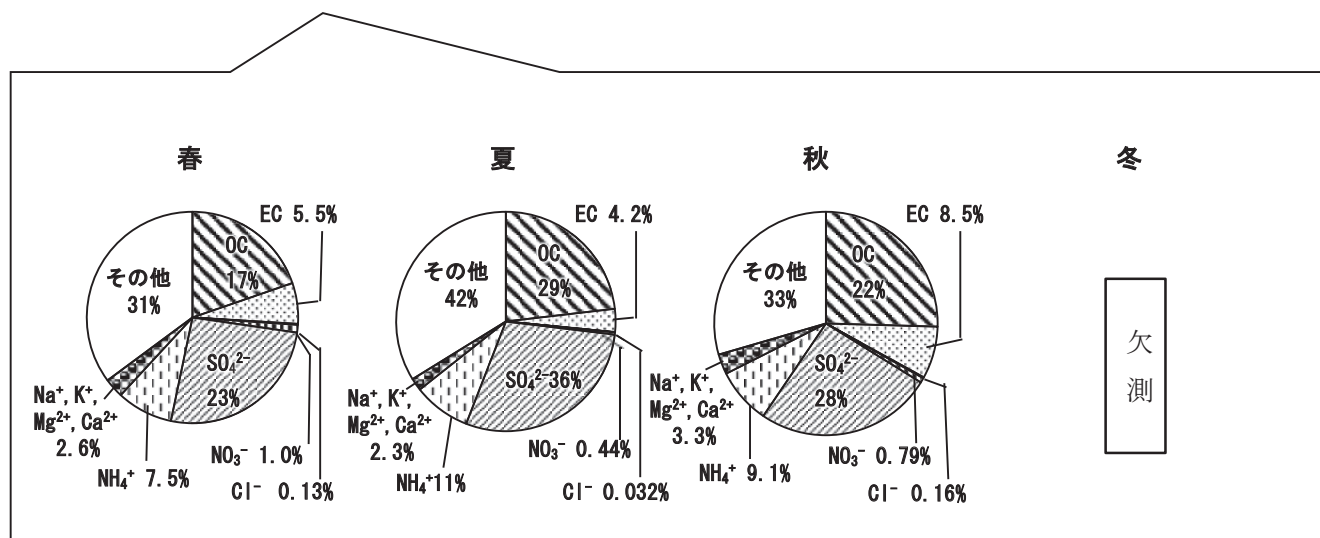
図3-7 PM2.5の成分組成（バックグラウンド）（令和5年度）
