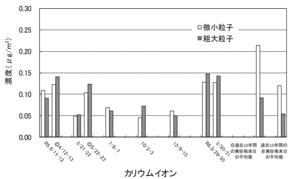
図7-4 粒径別イオン濃度
