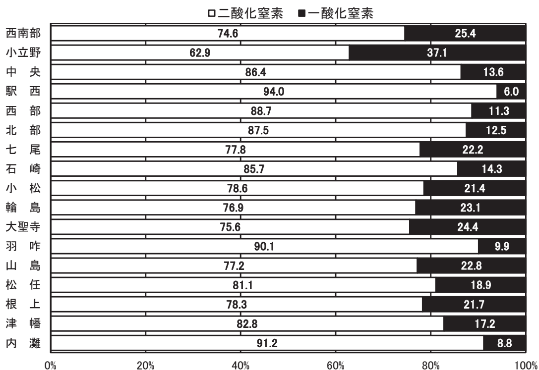
図 1－5 一般環境大気測定局における二酸化窒素と一酸化窒素の比率(令和 5 年度)
