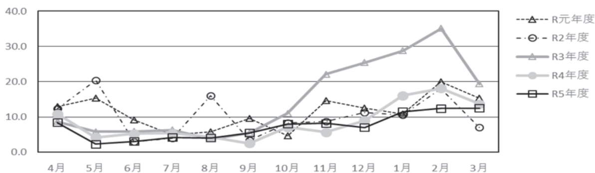
图 6-3 月別 nss- \text{SO}_4^{2-} 濃度
