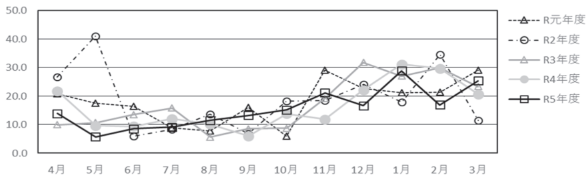
图 6-2 月別 \text{NO}_3^- 濃度
