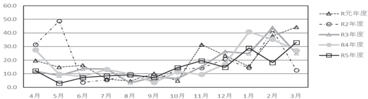
图 6-4 月別 \text{NH}_4^+ 濃度
