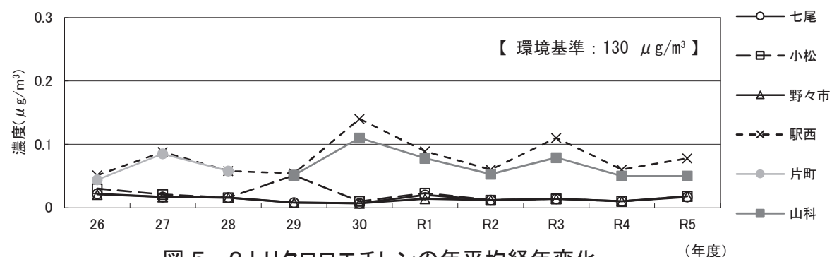
図5-2 トリクロロエチレンの年平均経年変化
