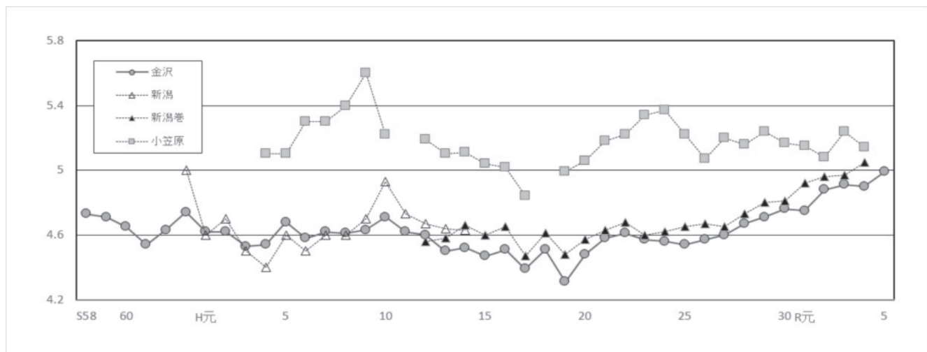
図 6－1 1 週間降水の pH(年平均値)の推移
