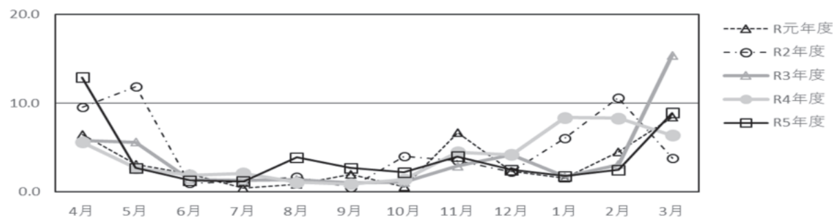
图 6-5 月別 nss- \text{Ca}^{2+} 濃度
