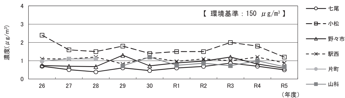
図 5-4 ジクロロメタンの経年変化
