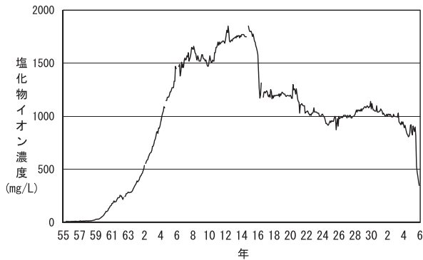
図5 能美市道林観測井の塩化物イオン濃度の経年変化（昭和56年～令和5年度）
