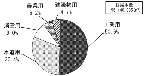
図6 用途別の地下水揚水量（令和4年度）
