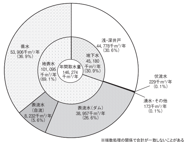
図10 水道水源別年間取水量(令和4年度)
