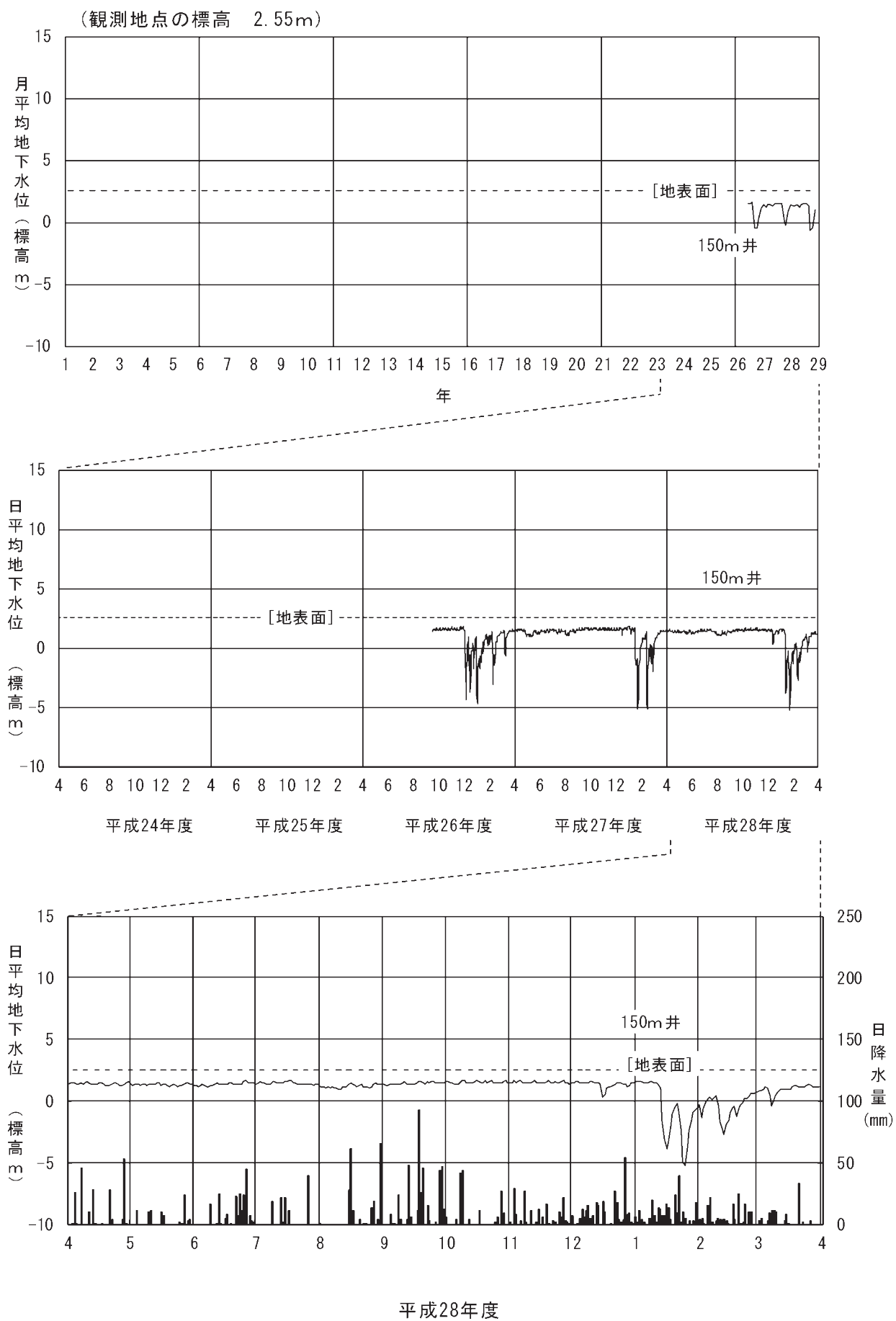
図 2-2-3(12) 地下水位 (⑫金沢市湊3丁目)
