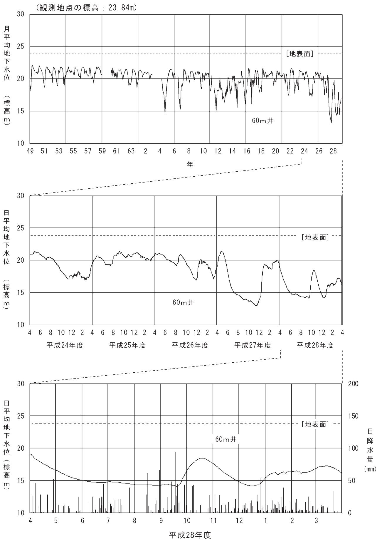
図 2-2-3(22) 地下水位 (㊸能美市北市)
