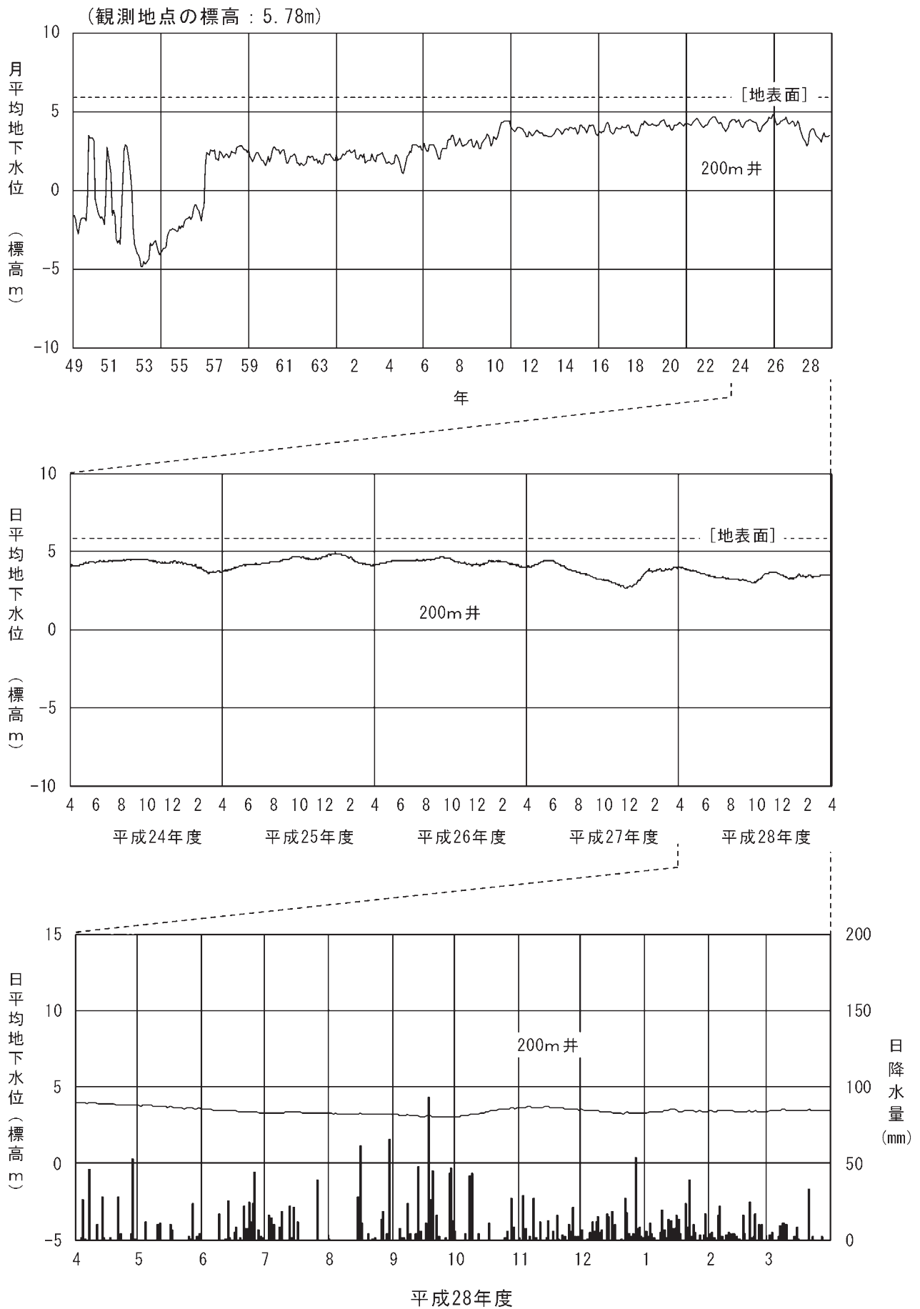
図 2-2-3(19) 地下水位 (㊟白山市井関)
