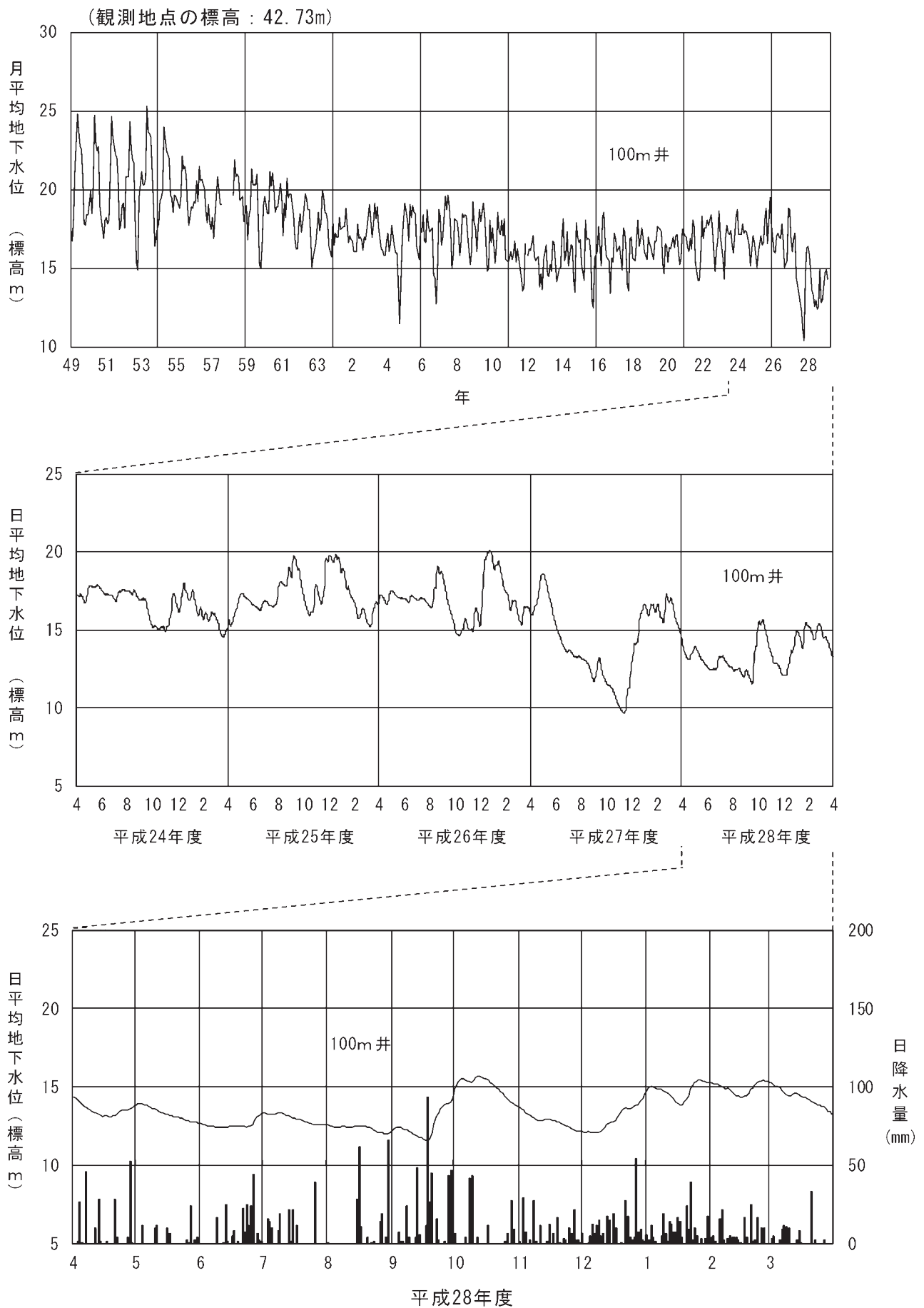
図 2-2-3 (20) 地下水位 (㊟白山市安吉町)
