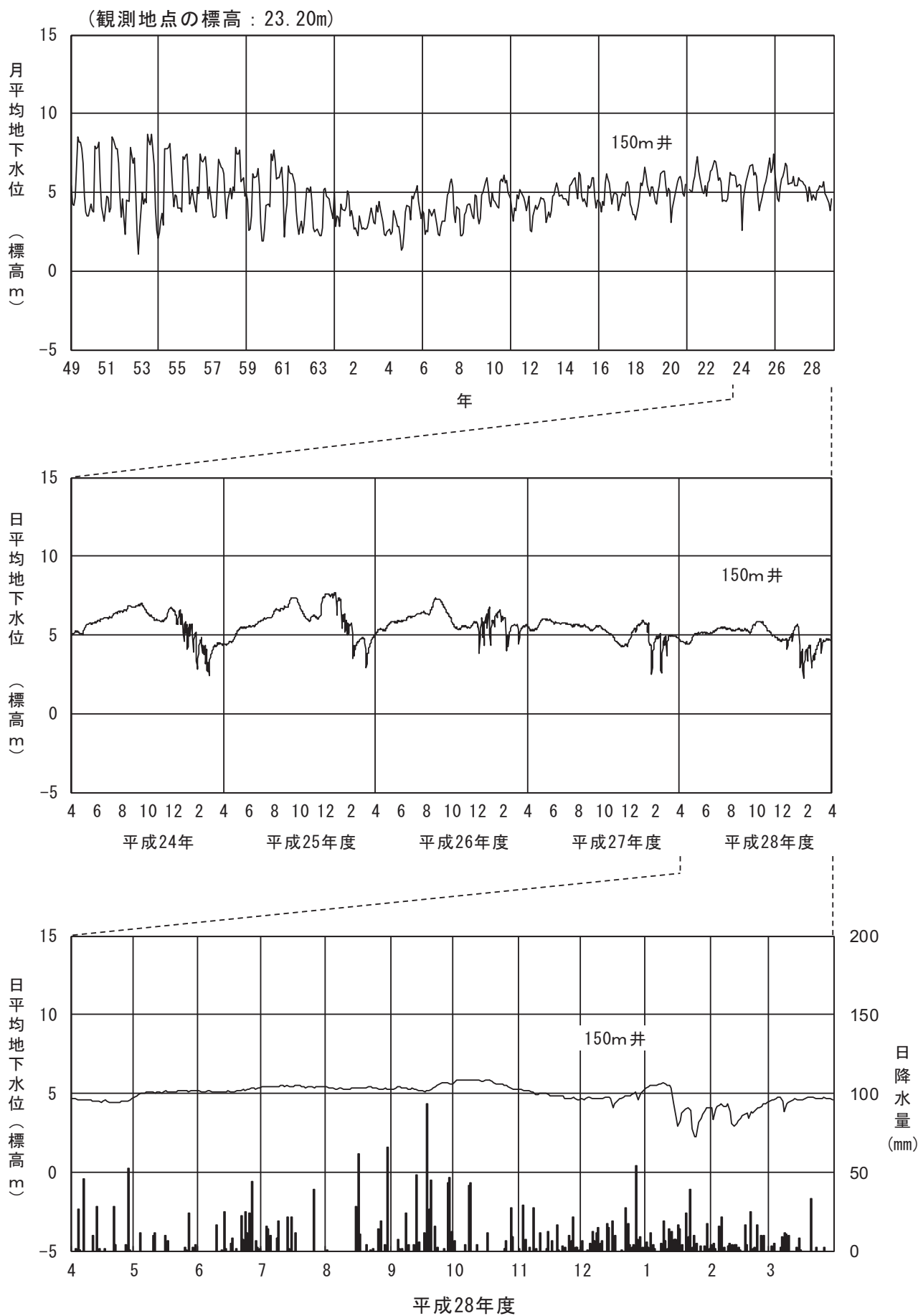
図 2-2-3(18) 地下水位 (⑱野々市市太平寺)
