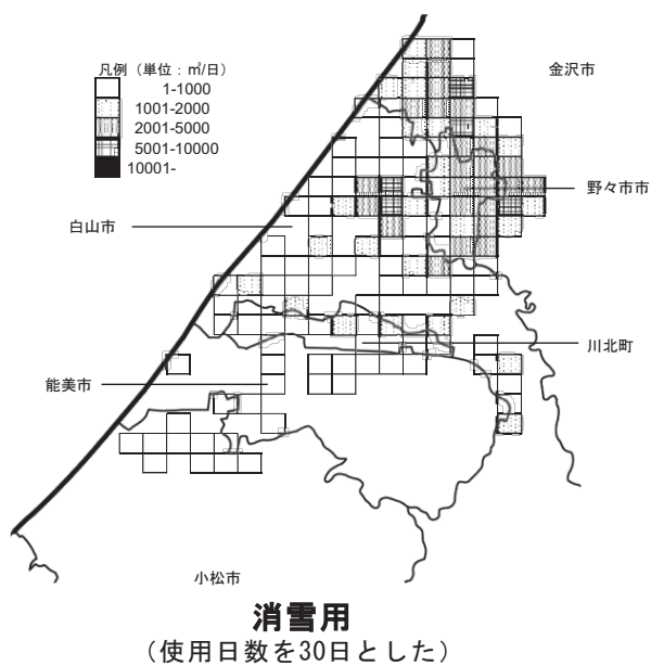
図 2-2-4 (3) メッシュ別の地下水揚水量 (平成 28 年度)
