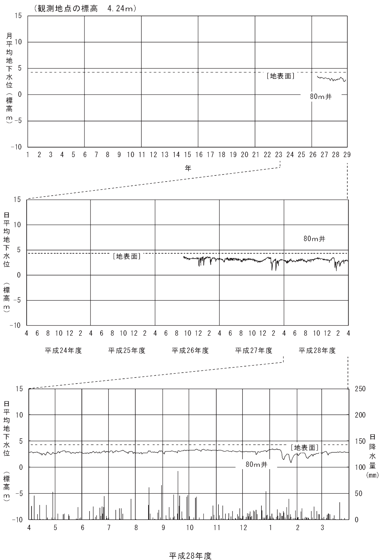
図 2-2-3(11) 地下水位 (⑪金沢市下安原町)
