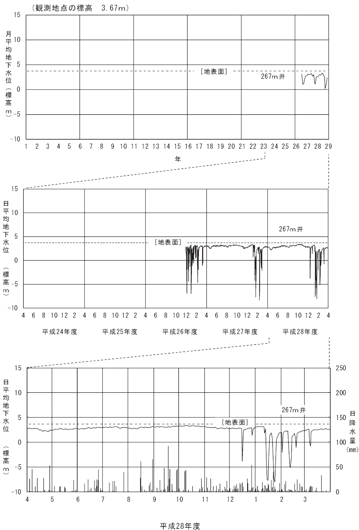
図 2-2-3(14) 地下水位 (⑭金沢市専光寺町)
