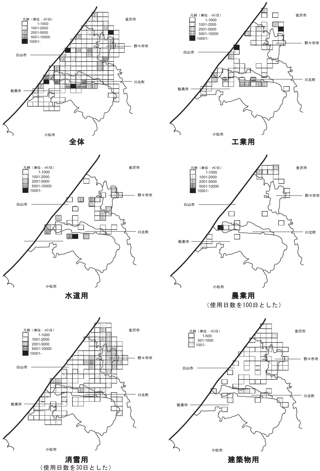
図 2-2-4(2) メッシュ別の地下水揚水量 (平成 27 年度)
