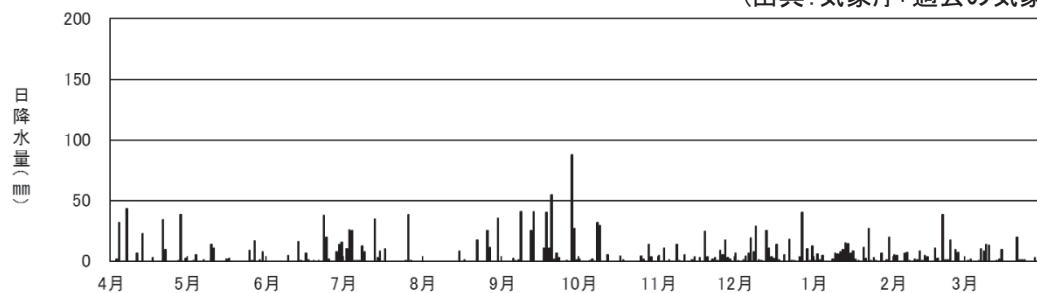
図 3-2-5 七尾地域気象観測所の日降水量 (平成 28 年度)
