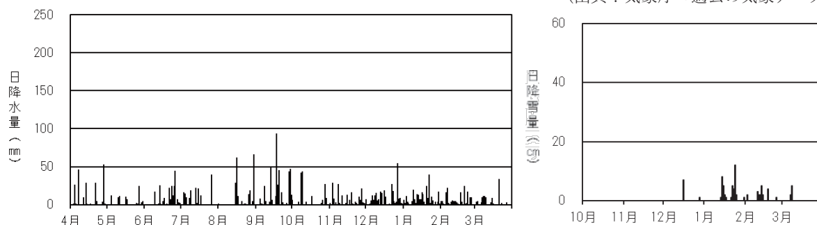
図 2-2-6 金沢地域気象観測所の日降水量と年間降雪量(平成 28 年度)
