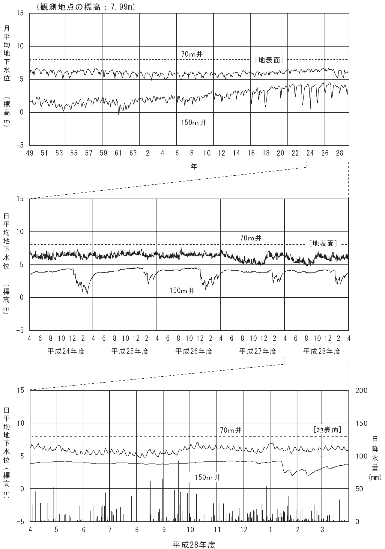
図 2-2-3(21) 地下水位 (㊴能美市赤井)
