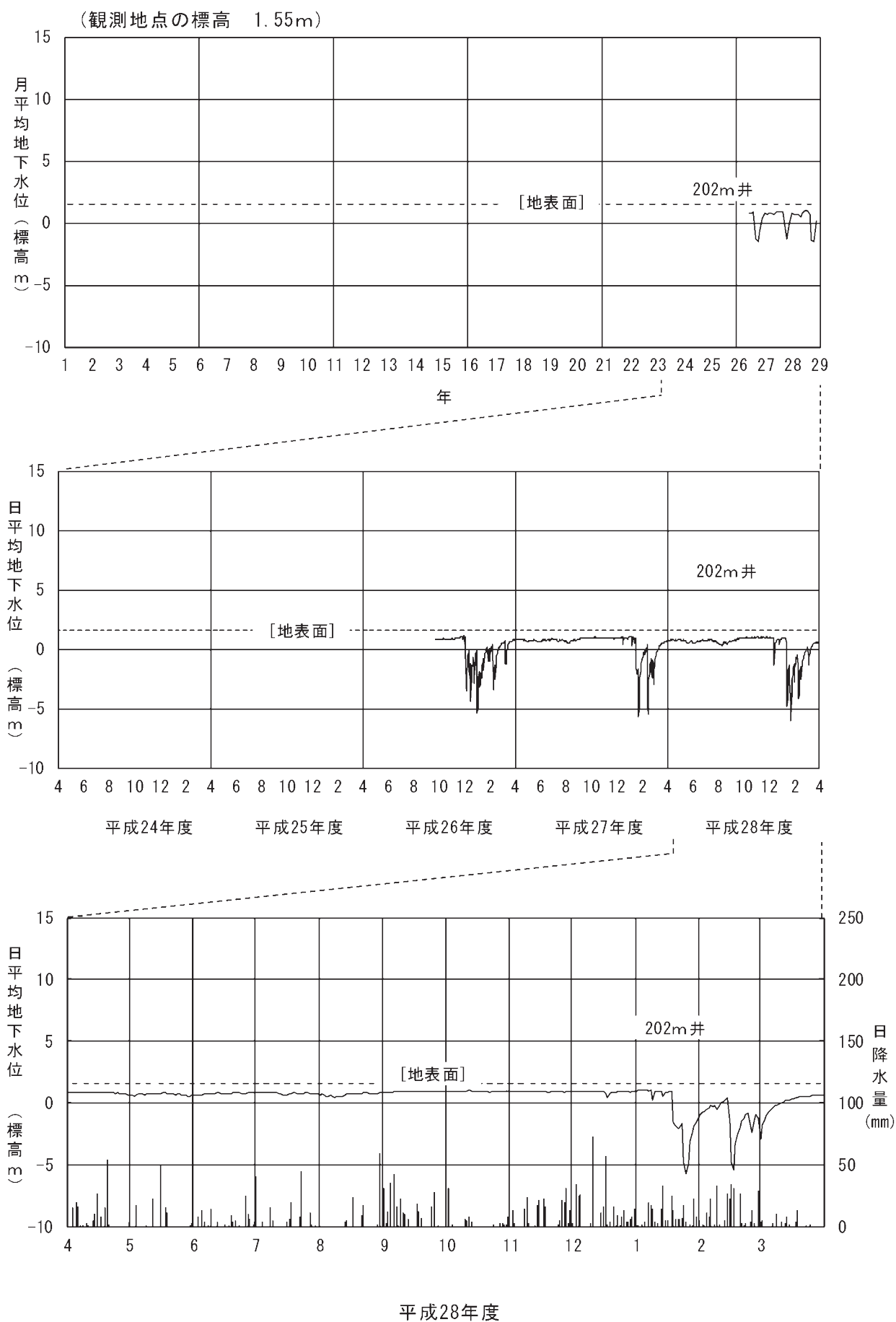
図 2-2-3(13) 地下水位 (⑬金沢市東蚊爪町)
