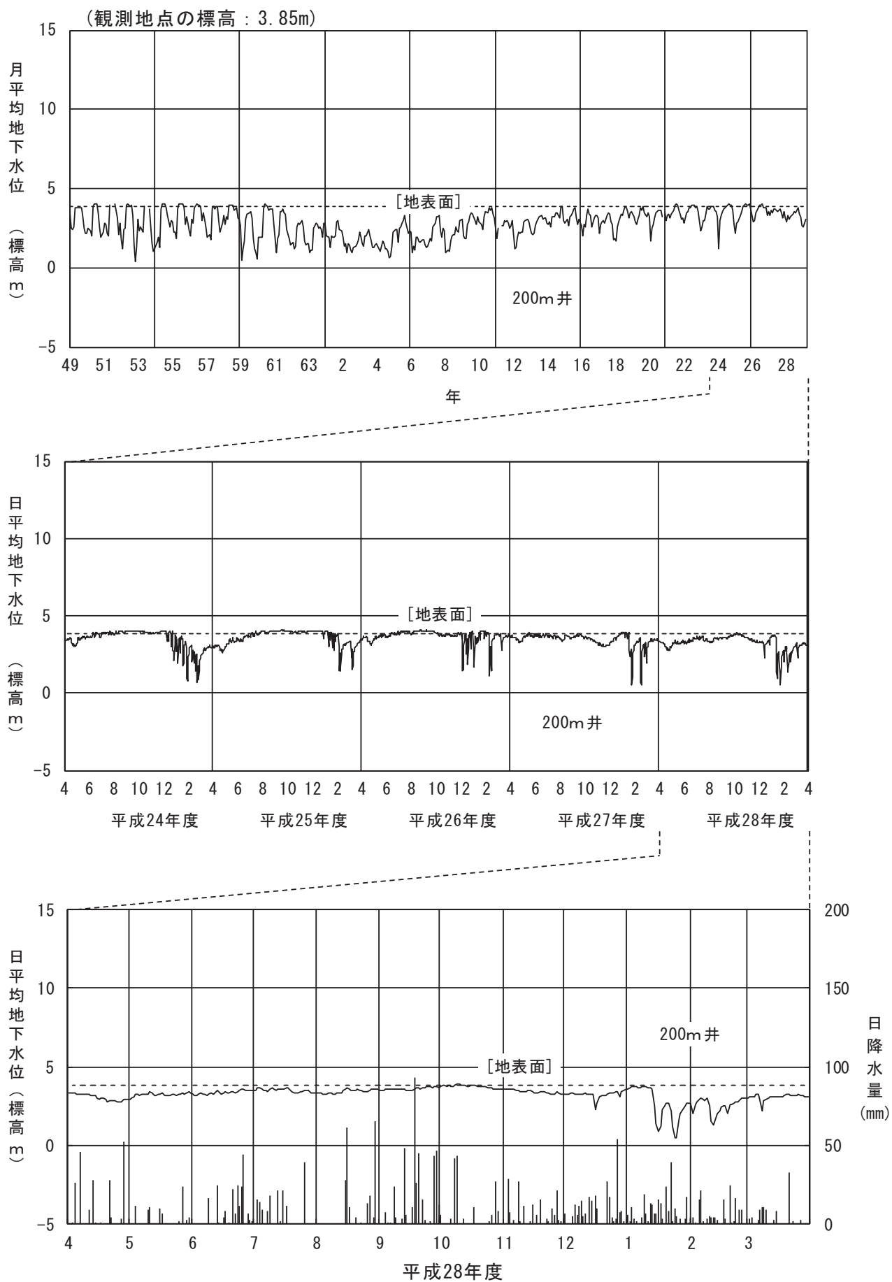
図 2-2-3 (15) 地下水位 (⑮金沢市福増町)
