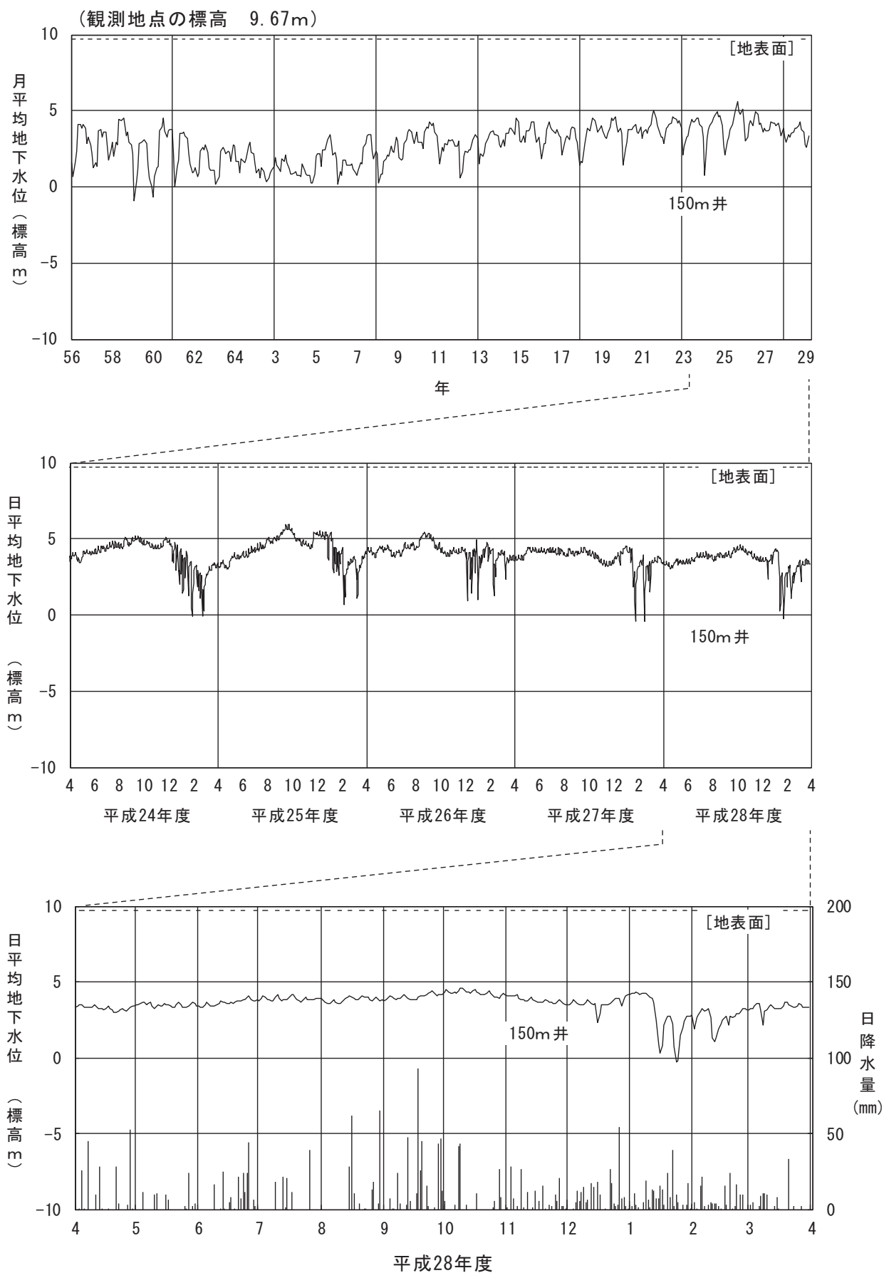
図 2-2-2 (9) 地下水位 (⑨金沢市新保本町)
