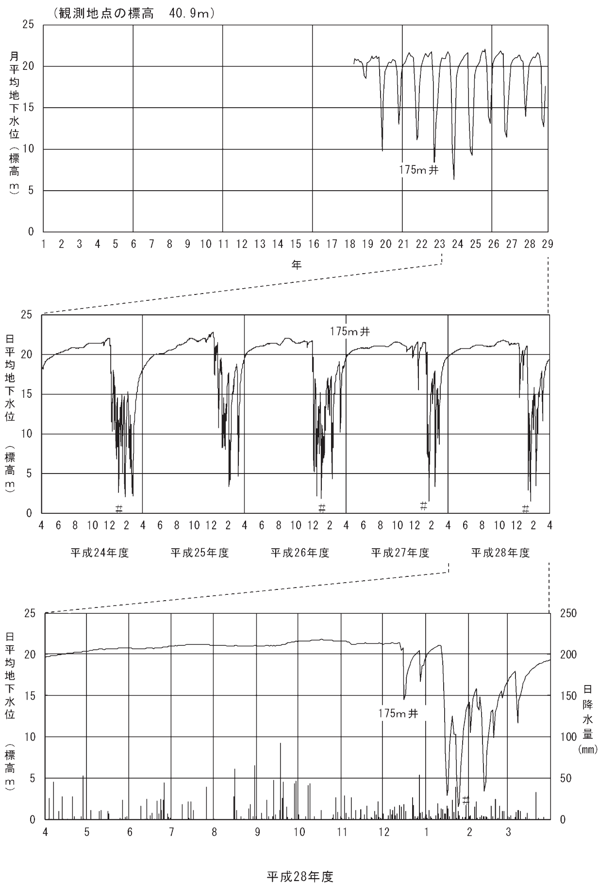
図 2-2-3(10) 地下水位 (⑩金沢市泉野出町)
