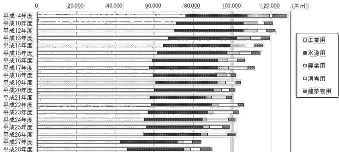
図 2-2-4(1) 用途別の地下水揚水量の経年変化
