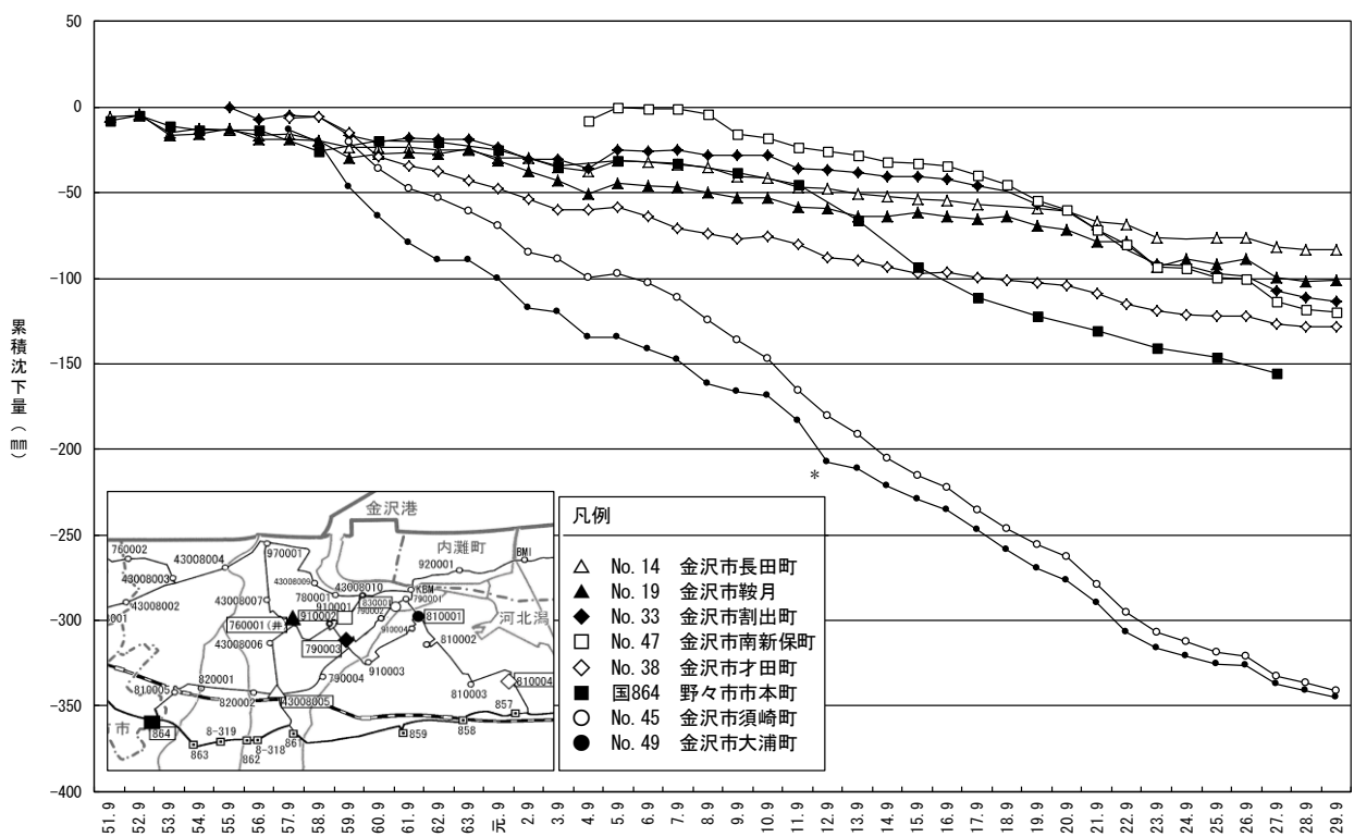
図 2-2-1(2) 主な水準点の累積地盤沈下量 (金沢市近郊)
