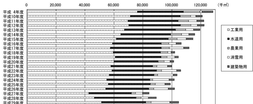
図 2-2-4(1) 用途別の地下水揚水量の経年変化
