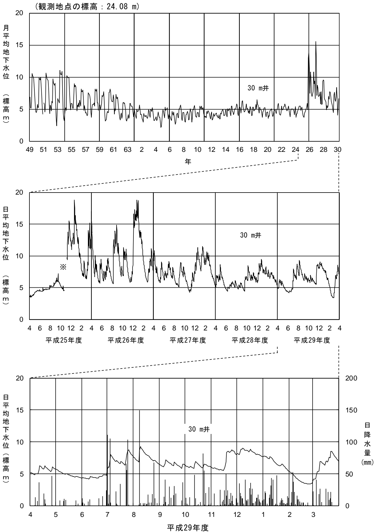
図 2-2-3(17) 地下水位 (①白山市末広)
