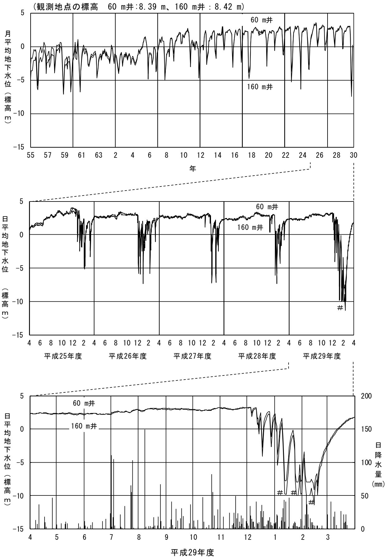
図 2-2-3 (3) 地下水位 (③金沢市浅野本町)
