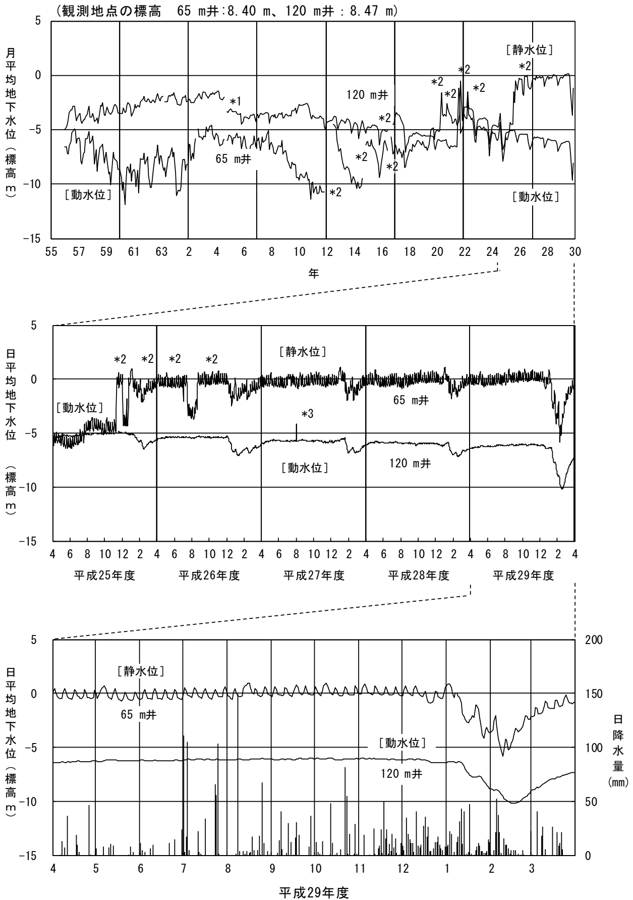
図 2-2-3 (23) 地下水位 (㊸能美市道林)
