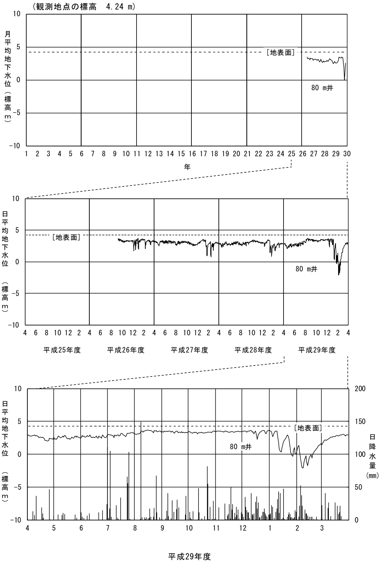
図 2-2-3(11) 地下水水位 (⑪金沢市下安原町)
