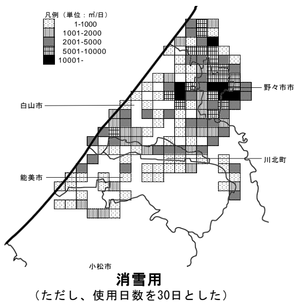
図 2-2-4 (2) メッシュ別の地下水揚水量 (平成 29 年度)
