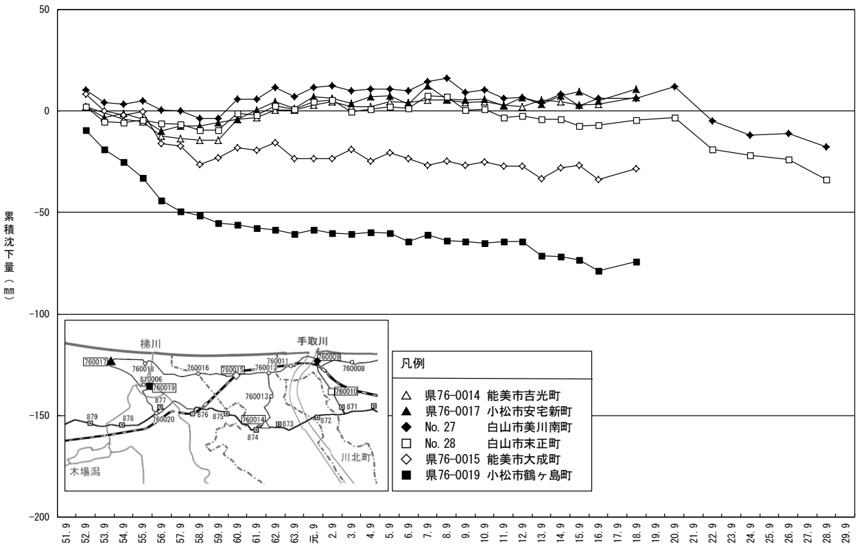
図 2-2-1 (4) 主な水準点の累積地盤沈下量 (白山市美川南町～小松市安宅新町)
