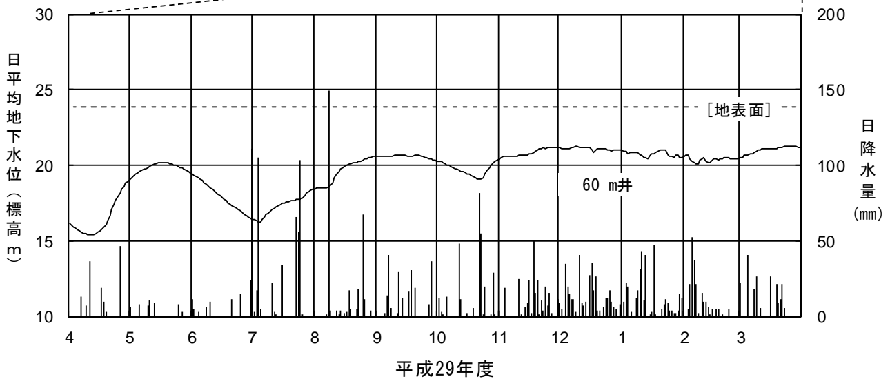
図 2-2-3 (22) 地下水位 (能美市北市)
