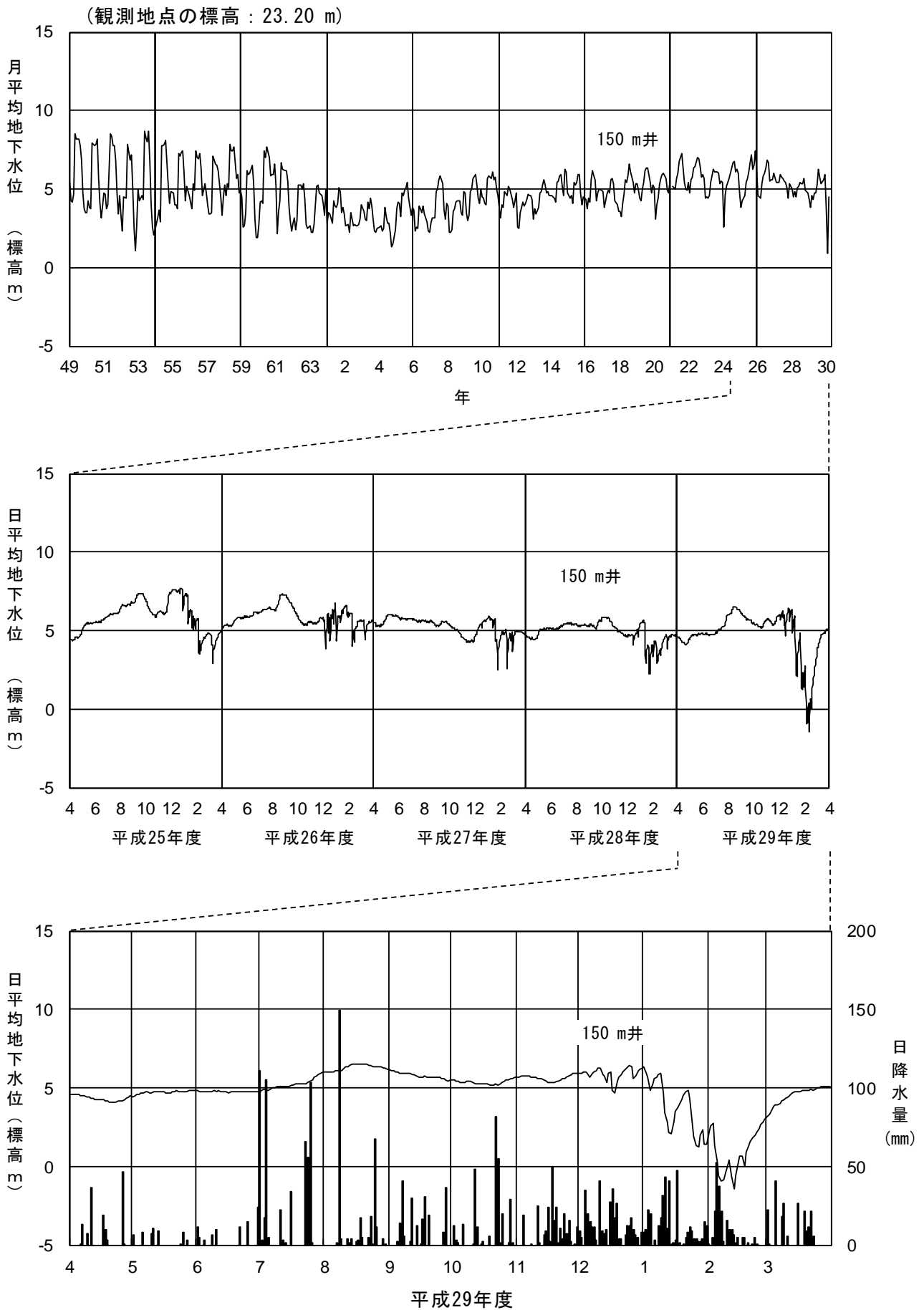
図 2-2-3(18) 地下水位 (野々市市太平寺)
