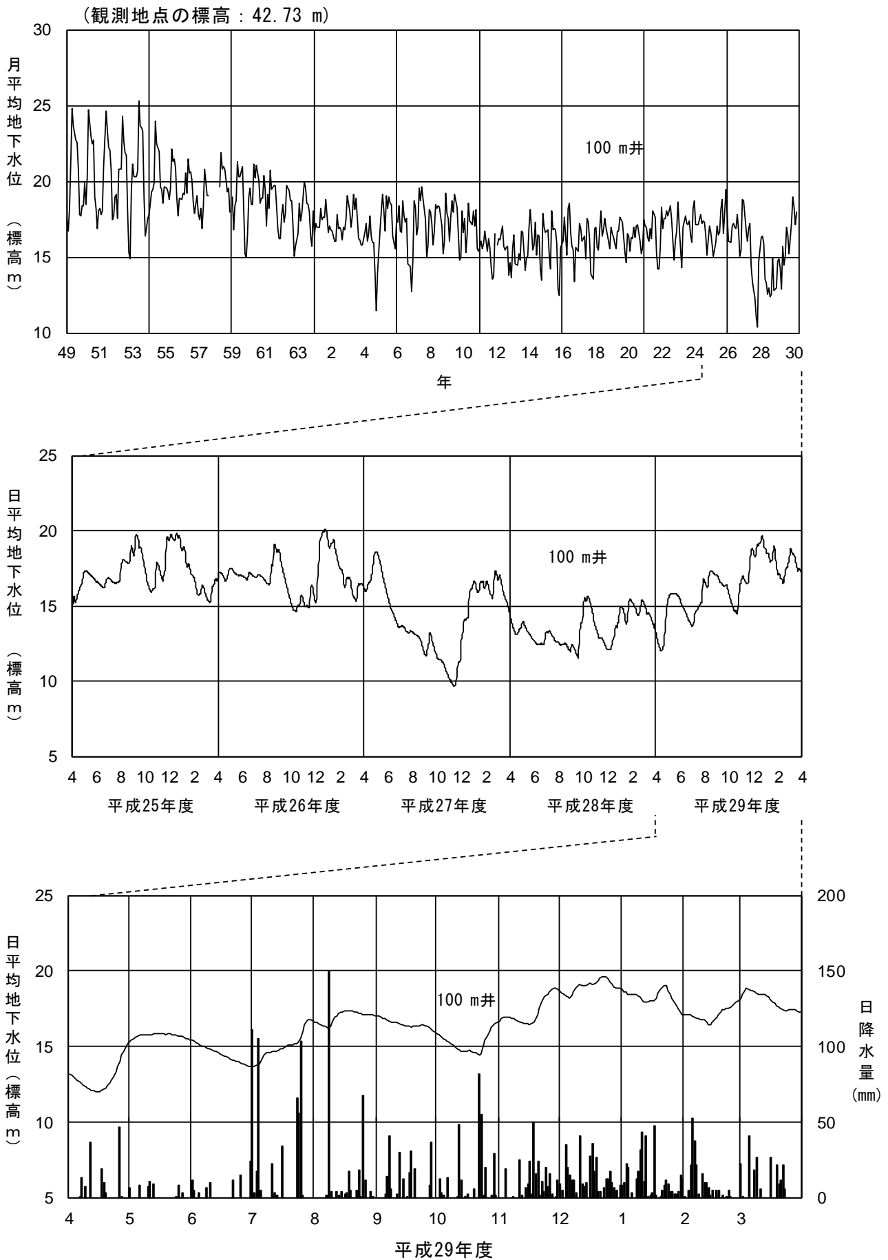
図 2-2-3 (20) 地下水位 (㊸白山市安吉町)
