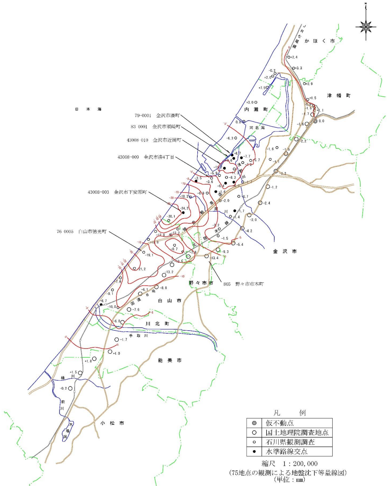
図2-2-1(5) 地盤沈下等量線図(平成27年9月～平成29年9月)
