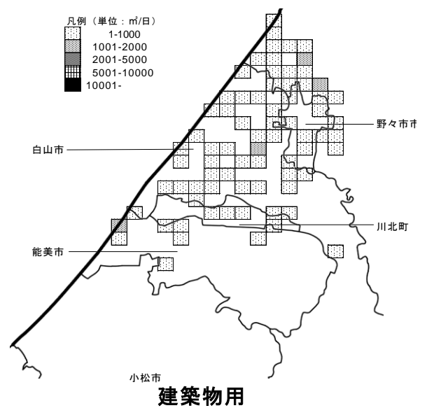
図 2-2-4 (2) メッシュ別の地下水揚水量 (平成 29 年度)
