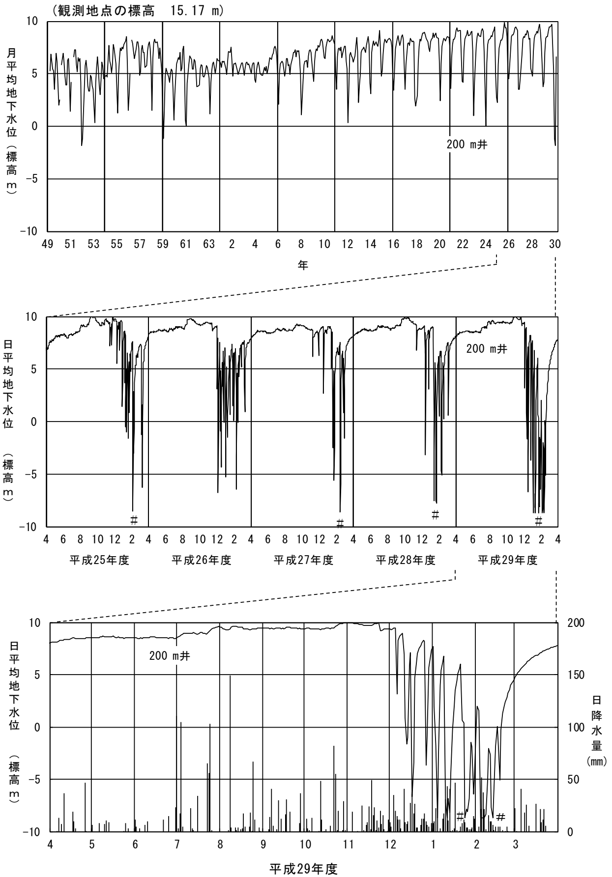
図 2-2-3(8) 地下水位 (⑧金沢市長町)
