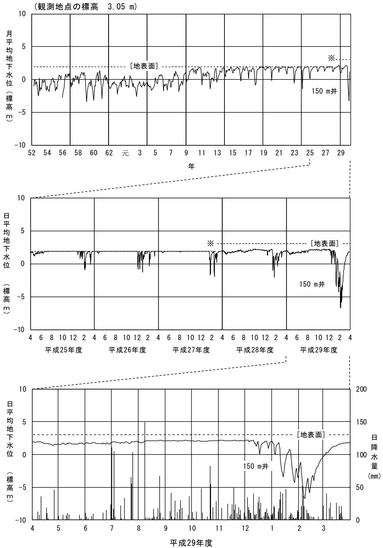
※井戸の改修に伴い、基準点が変更となり、標高が変化した(平成 28 年 3 月) 図 2-2-3(5) 地下水水位 (⑤金沢市金石東)
