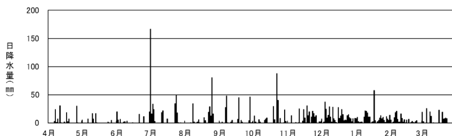
図3-2-5 七尾地域気象観測所の日降水量(平成29年度)
