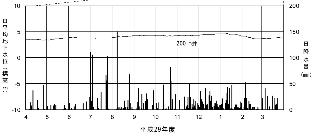
図 2-2-3(19) 地下水位 (㊟白山市井関)
