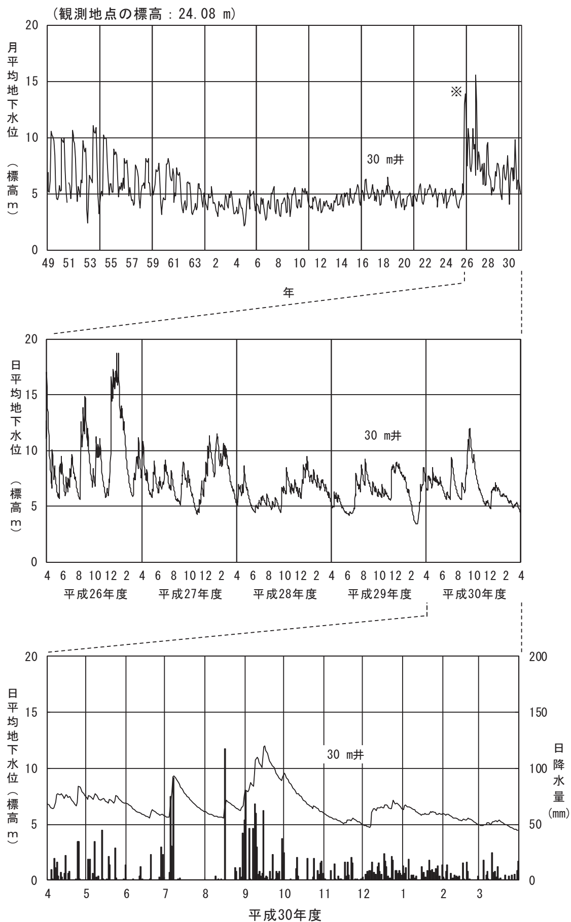
図 2-2-3 (17) 地下水位 (①白山市末広)
