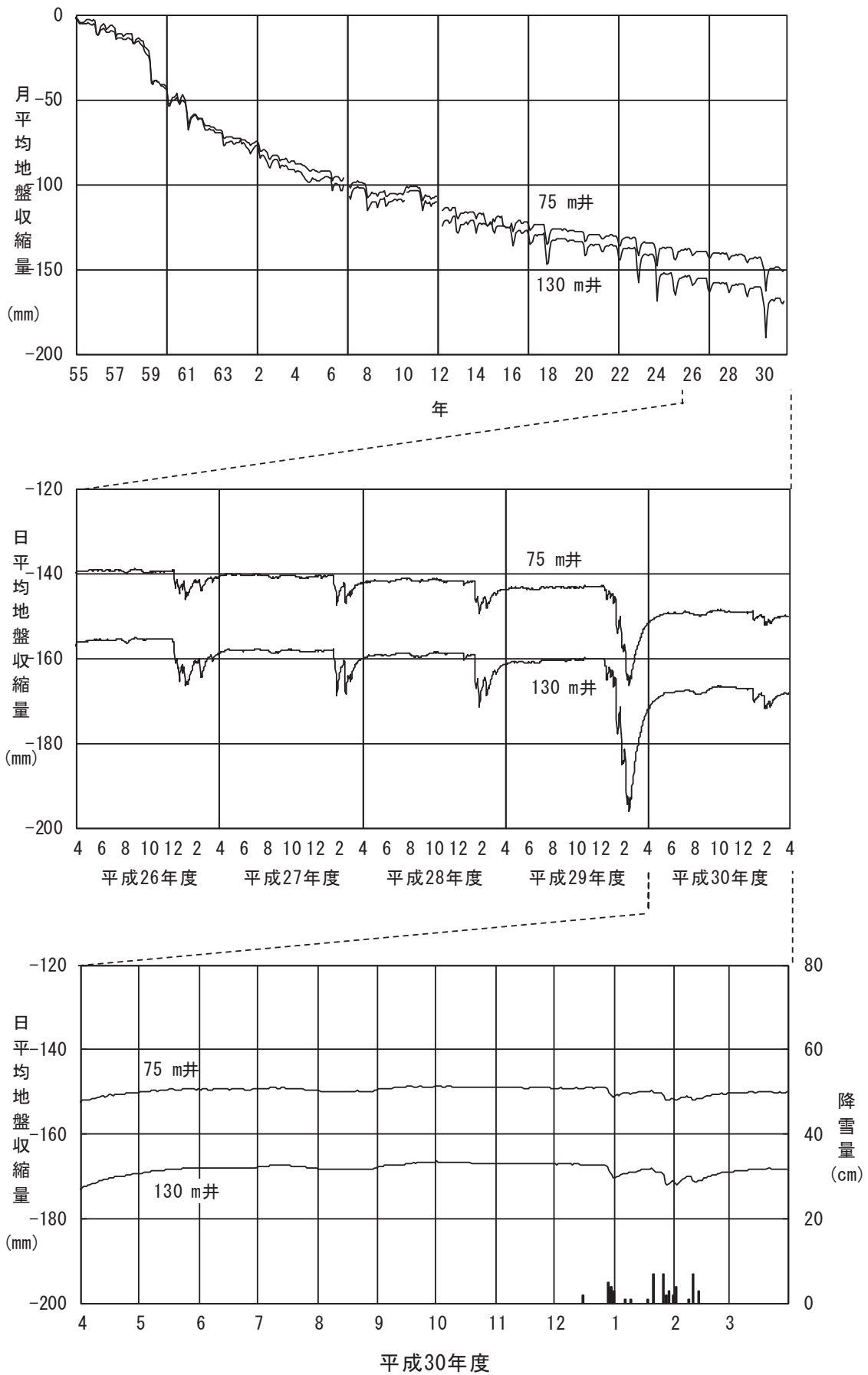
図 2-2-2(2) 地盤収縮量 (②金沢市須崎町)
