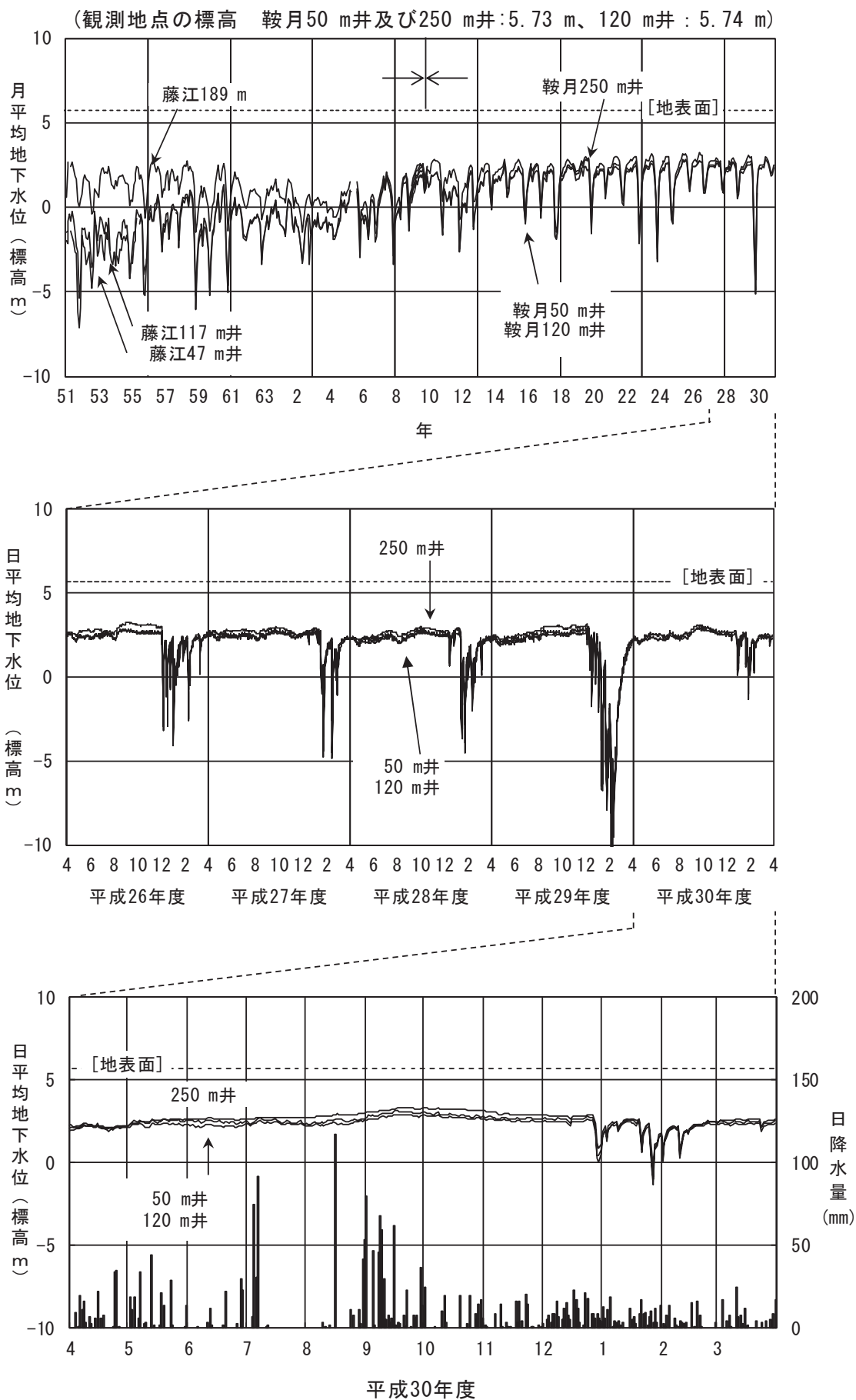
図 2-2-3(1) 地下水位 (①金沢市鞍月)
