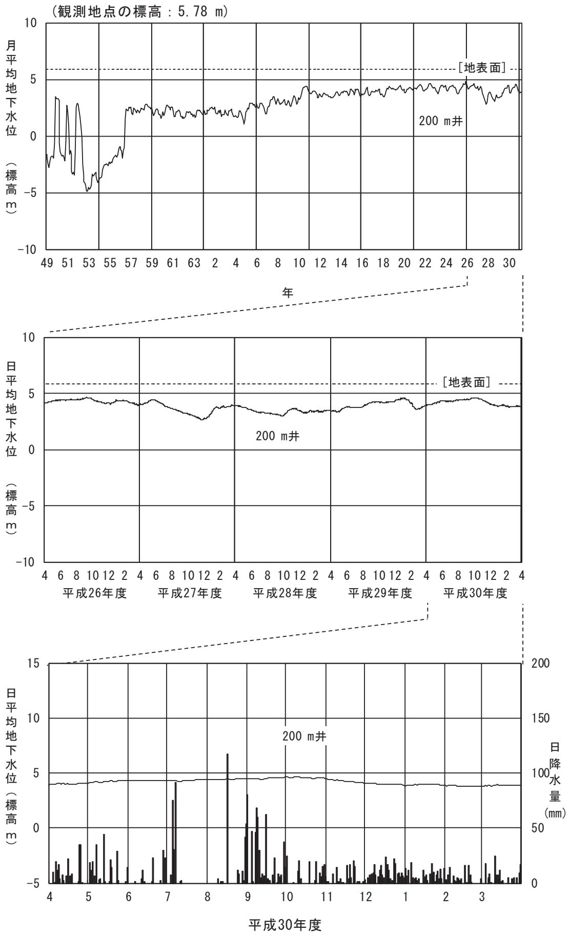
図 2-2-3(19) 地下水位 (㊟白山市井関)
