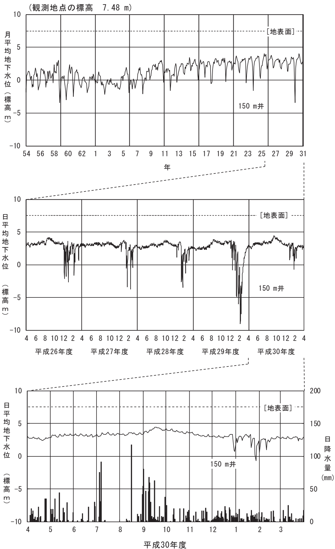
図 2-2-3(4) 地下水位 (④金沢市東力町)
