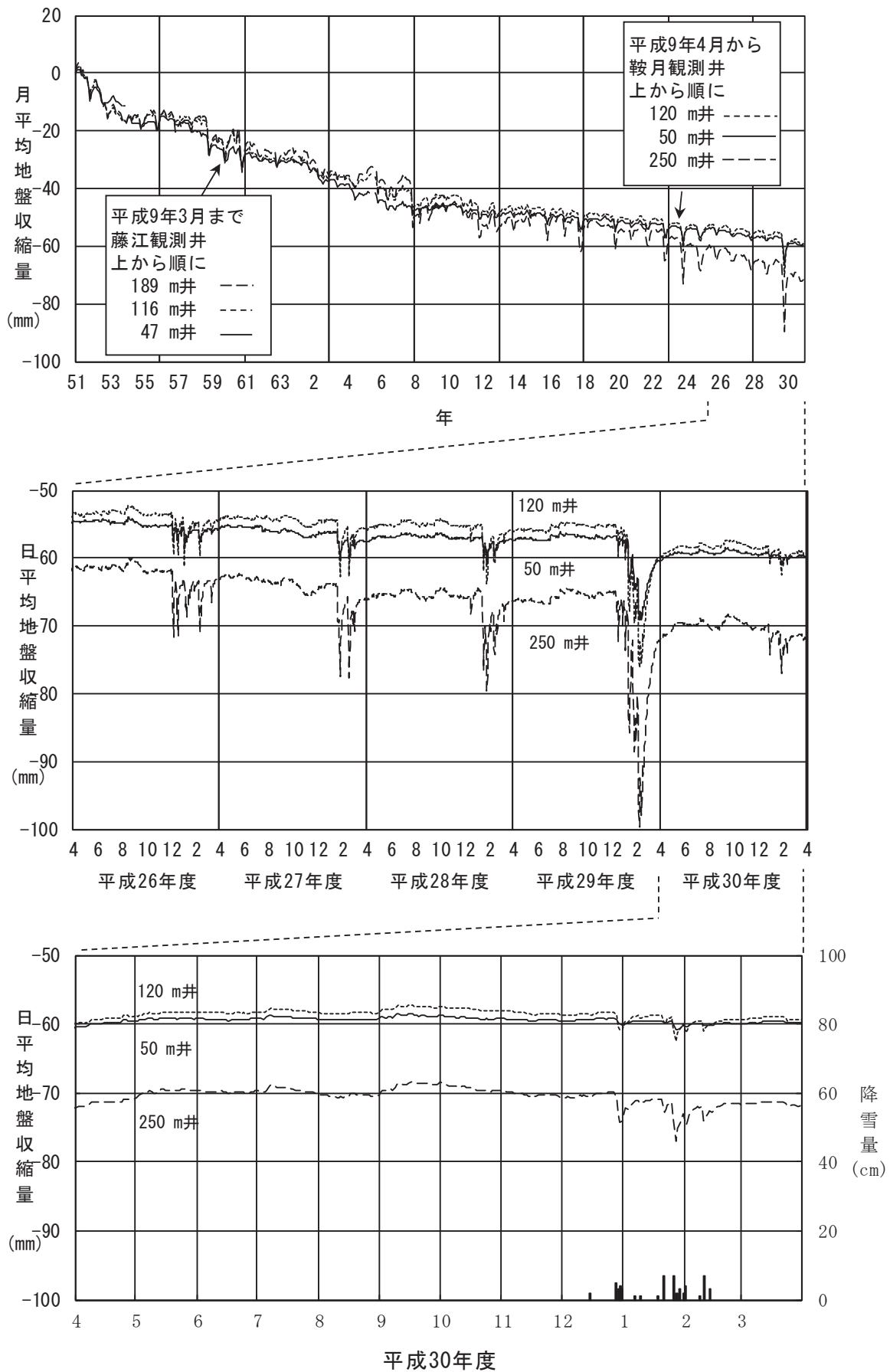
図 2-2-2(1) 地盤収縮量 (①金沢市鞍月)
