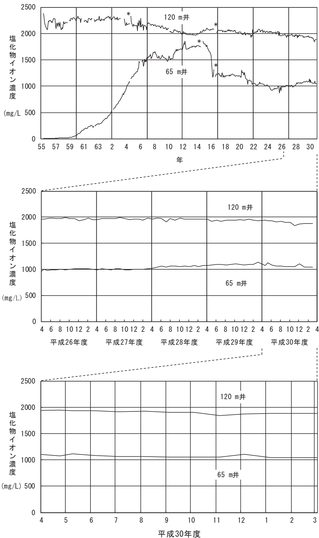
図 2-2-5 地下水質（塩化物イオン濃度）（㊸能美市道林）
