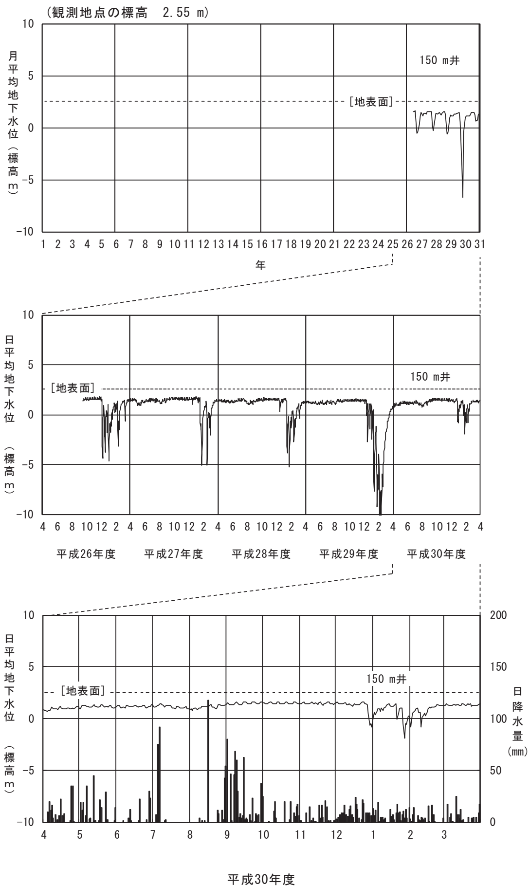
図 2-2-3(12) 地下水位 (⑫金沢市湊3丁目)
