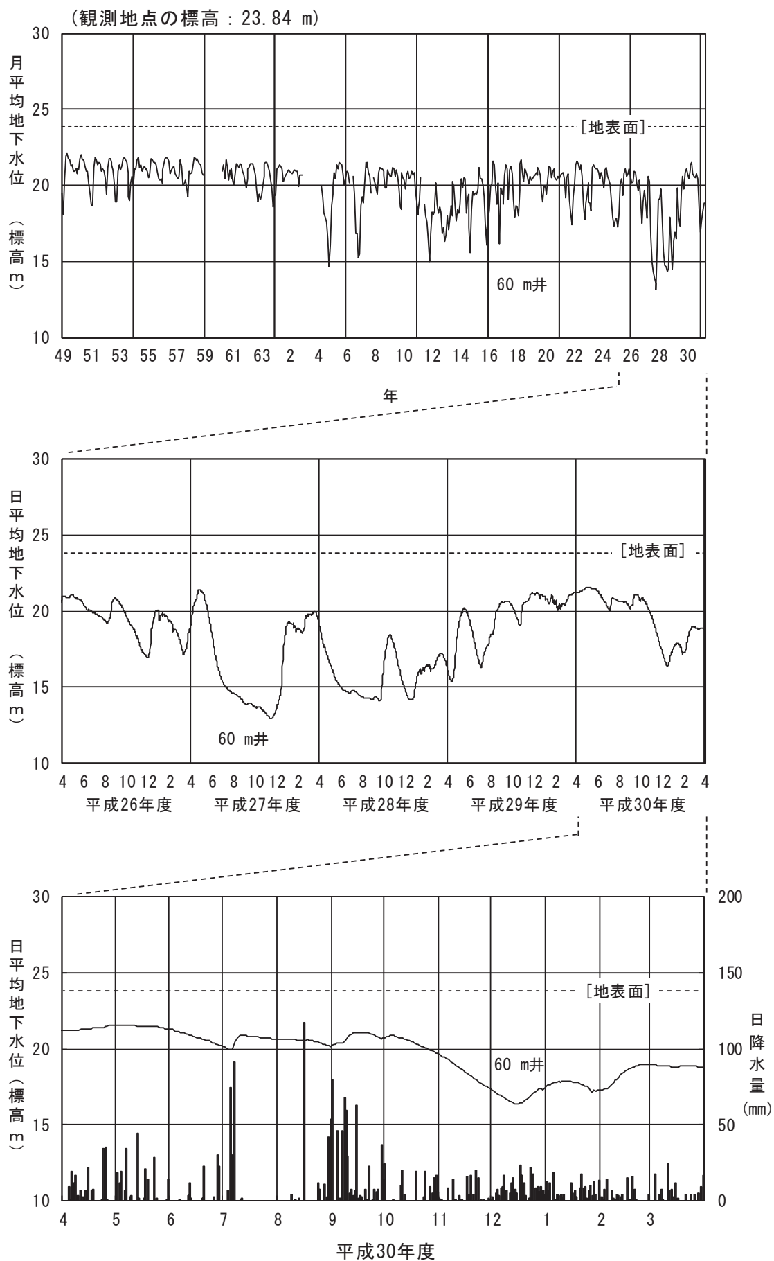
図 2-2-3 (22) 地下水位 (能美市北市)
