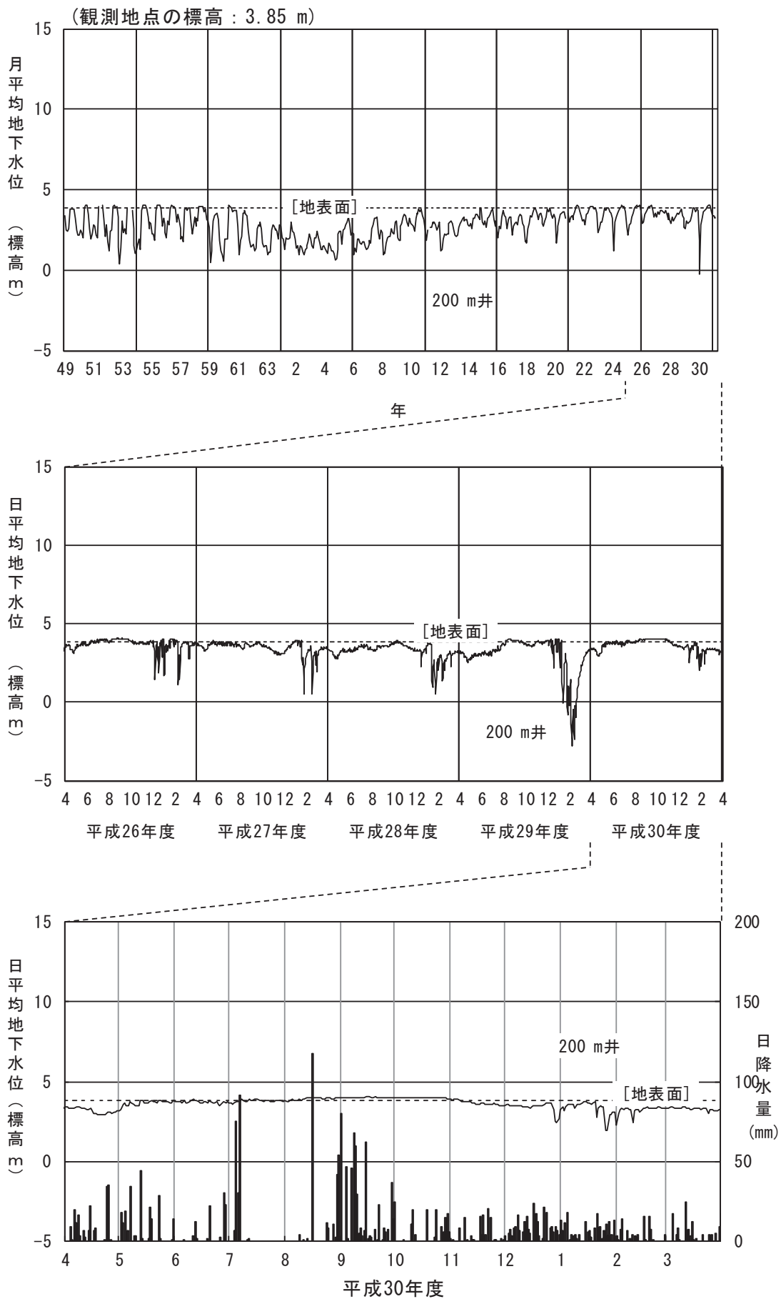
図 2-2-3(15) 地下水位 (⑮金沢市福増町)
