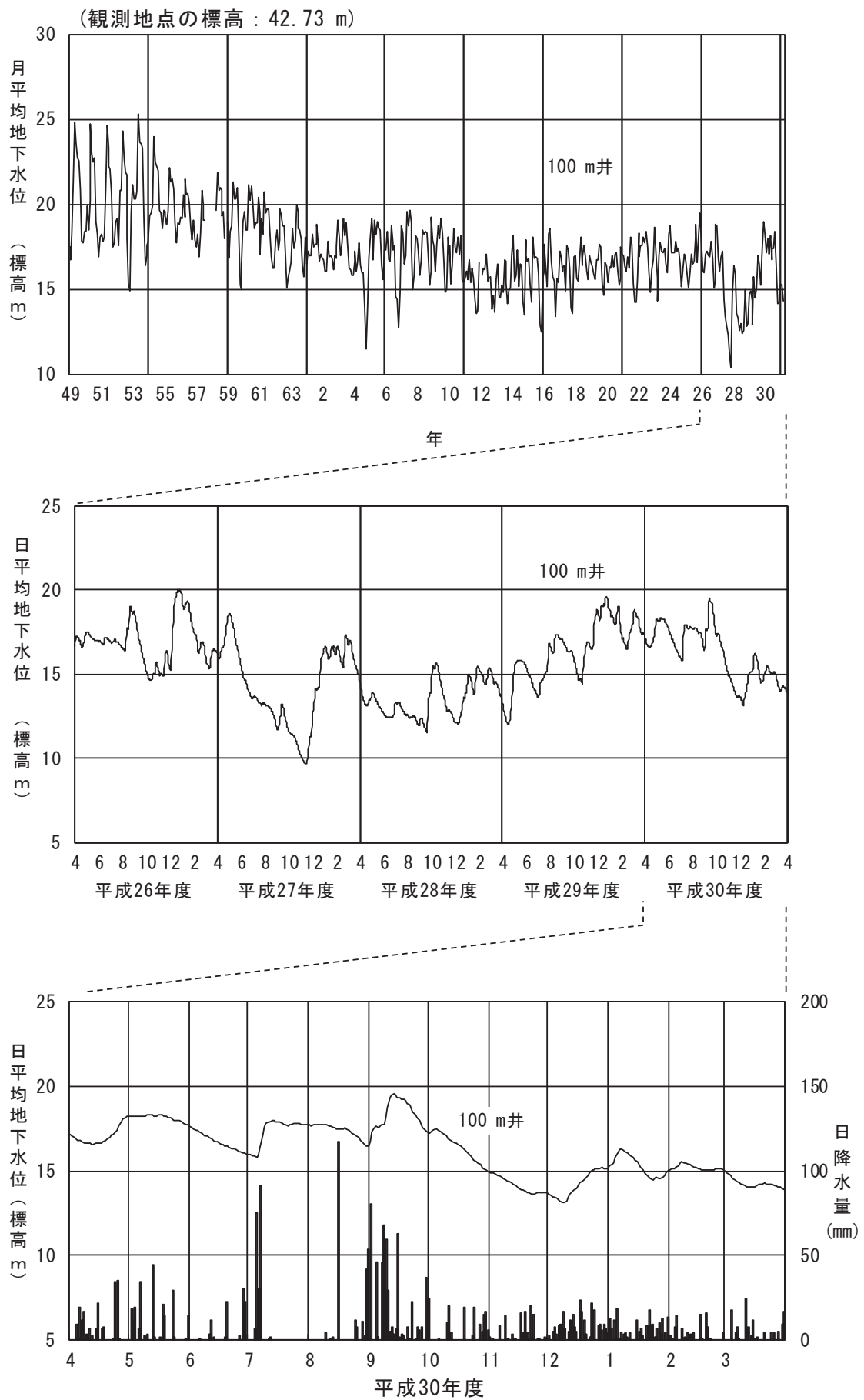
図 2-2-3(20) 地下水位 (㊸白山市安吉町)
