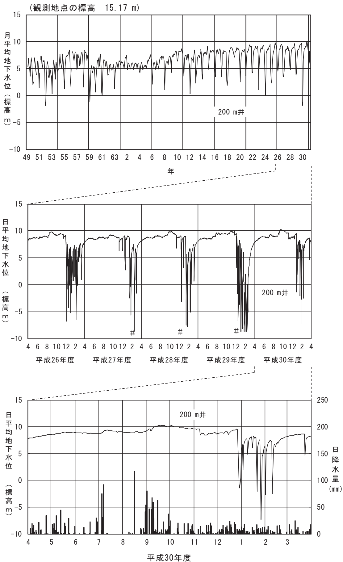
図 2-2-3(8) 地下水位 (⑧金沢市長町)
