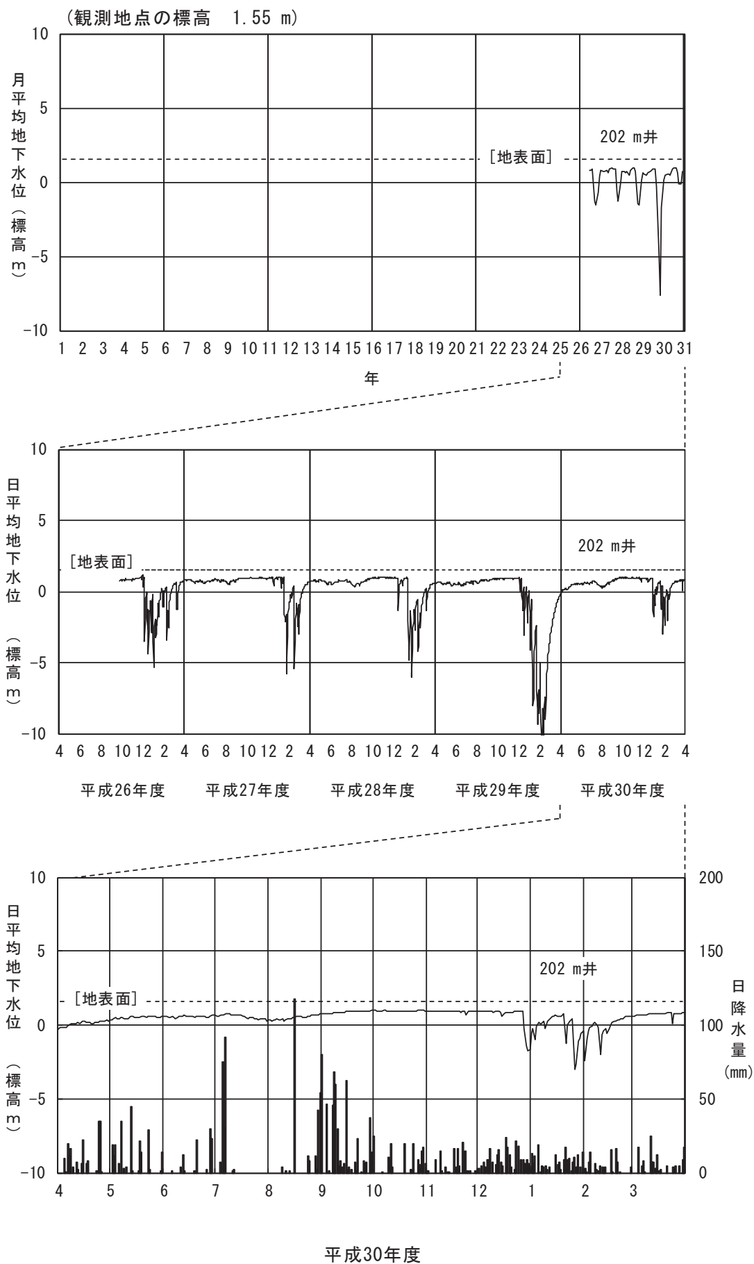
図 2-2-3(13) 地下水位 (⑬金沢市東蚊爪町)
