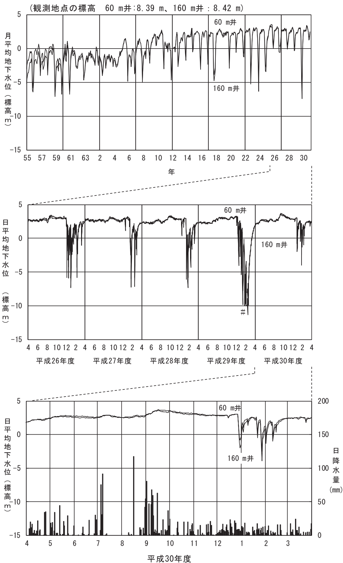
図 2-2-3 (3) 地下水位 (③金沢市浅野本町)
