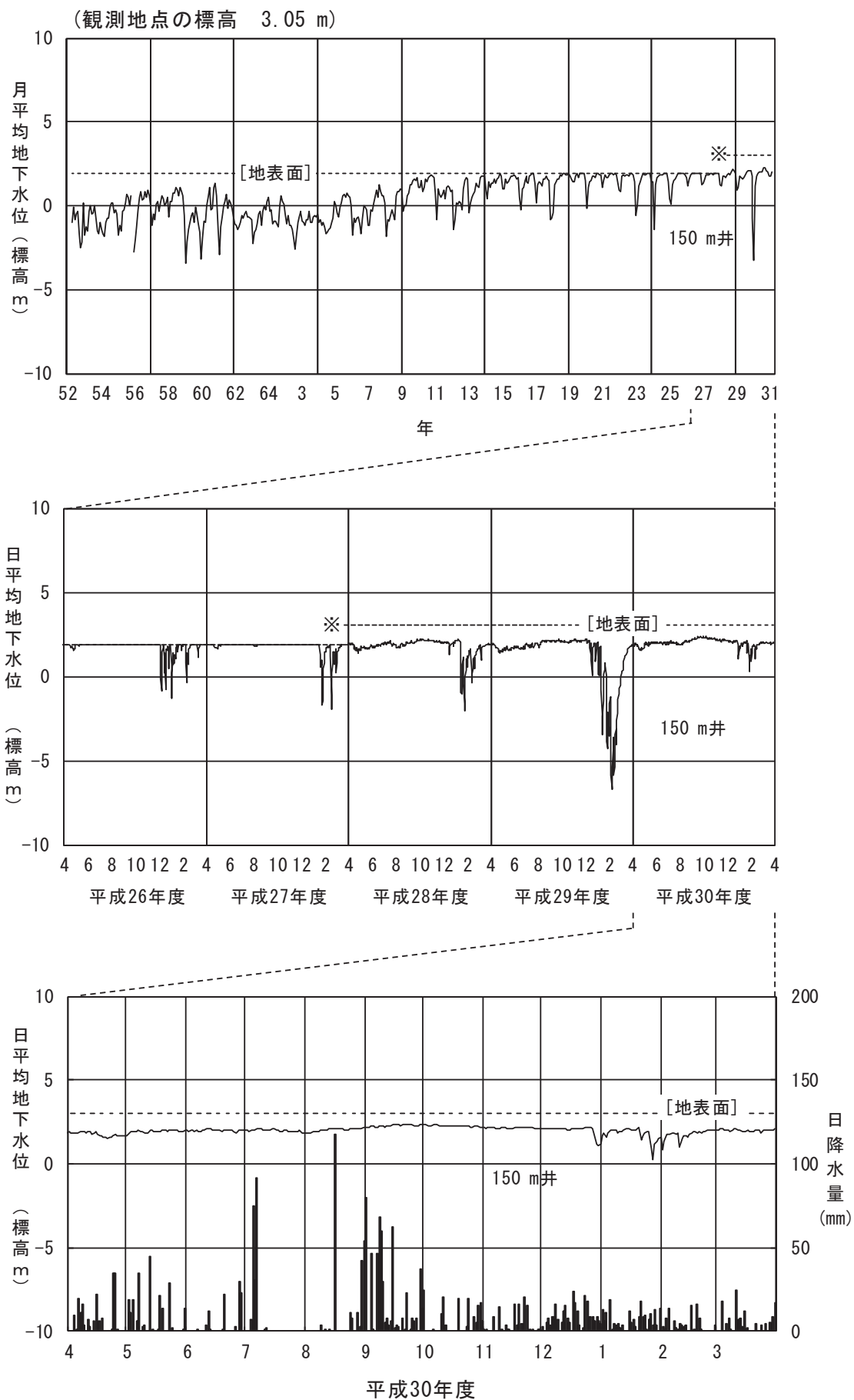
図 2-2-3(5) 地下水位 (⑤金沢市金石東)
