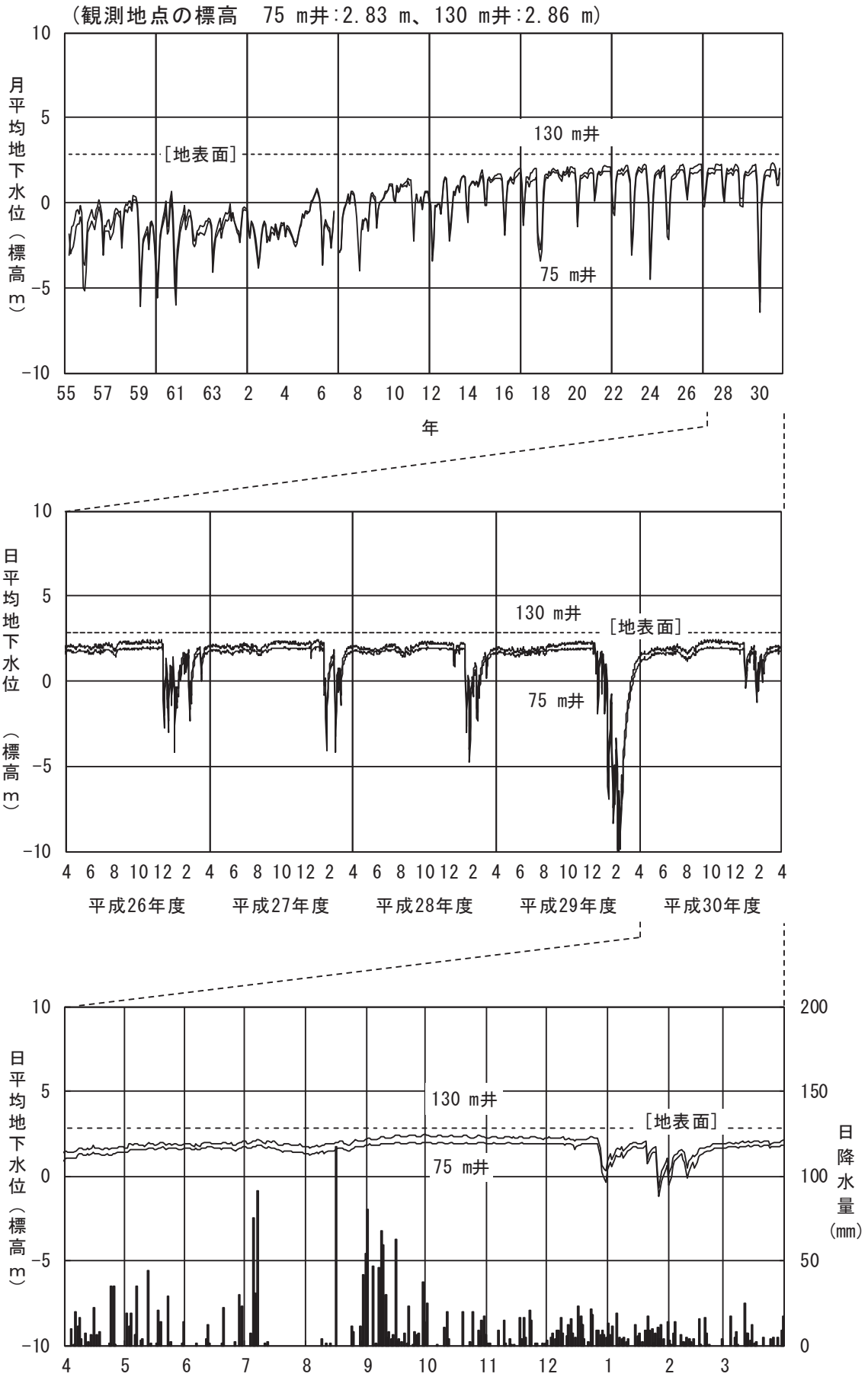
図 2-2-3 (2) 地下水位 (②金沢市須崎町)
