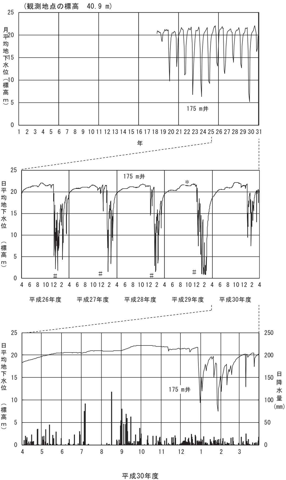
図 2-2-3(10) 地下水位 (⑩金沢市泉野出町)
