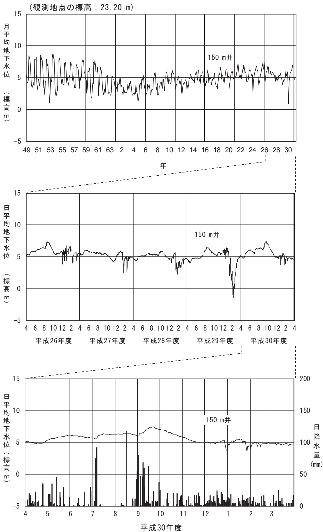
図 2-2-3(18) 地下水位 (⑱野々市市太平寺)
