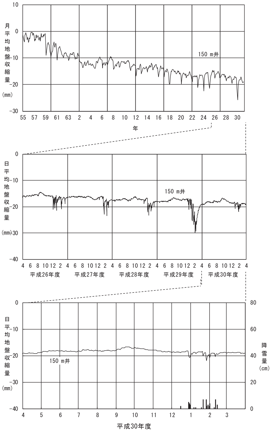
図 2-2-2(4) 地盤収縮量 (④金沢市東力町)
