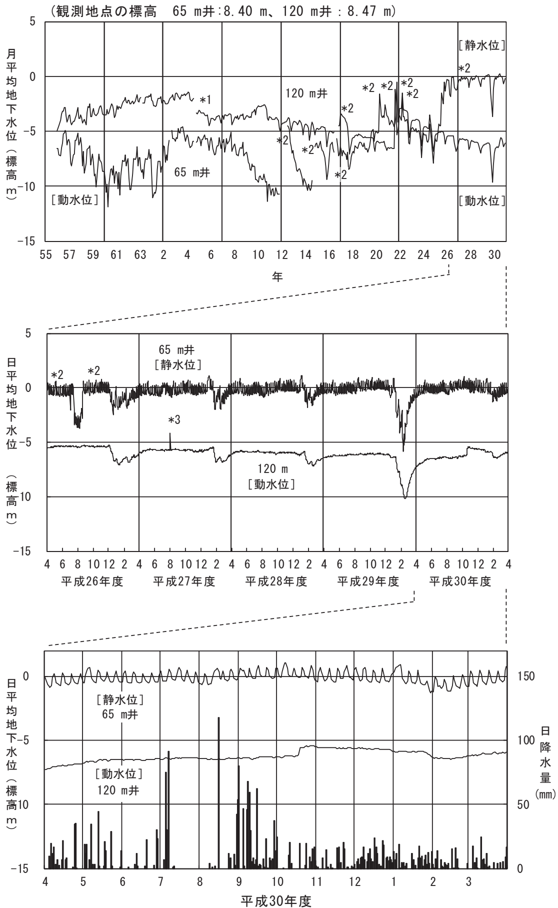
図 2-2-3 (23) 地下水水位 (㊸能美市道林)
