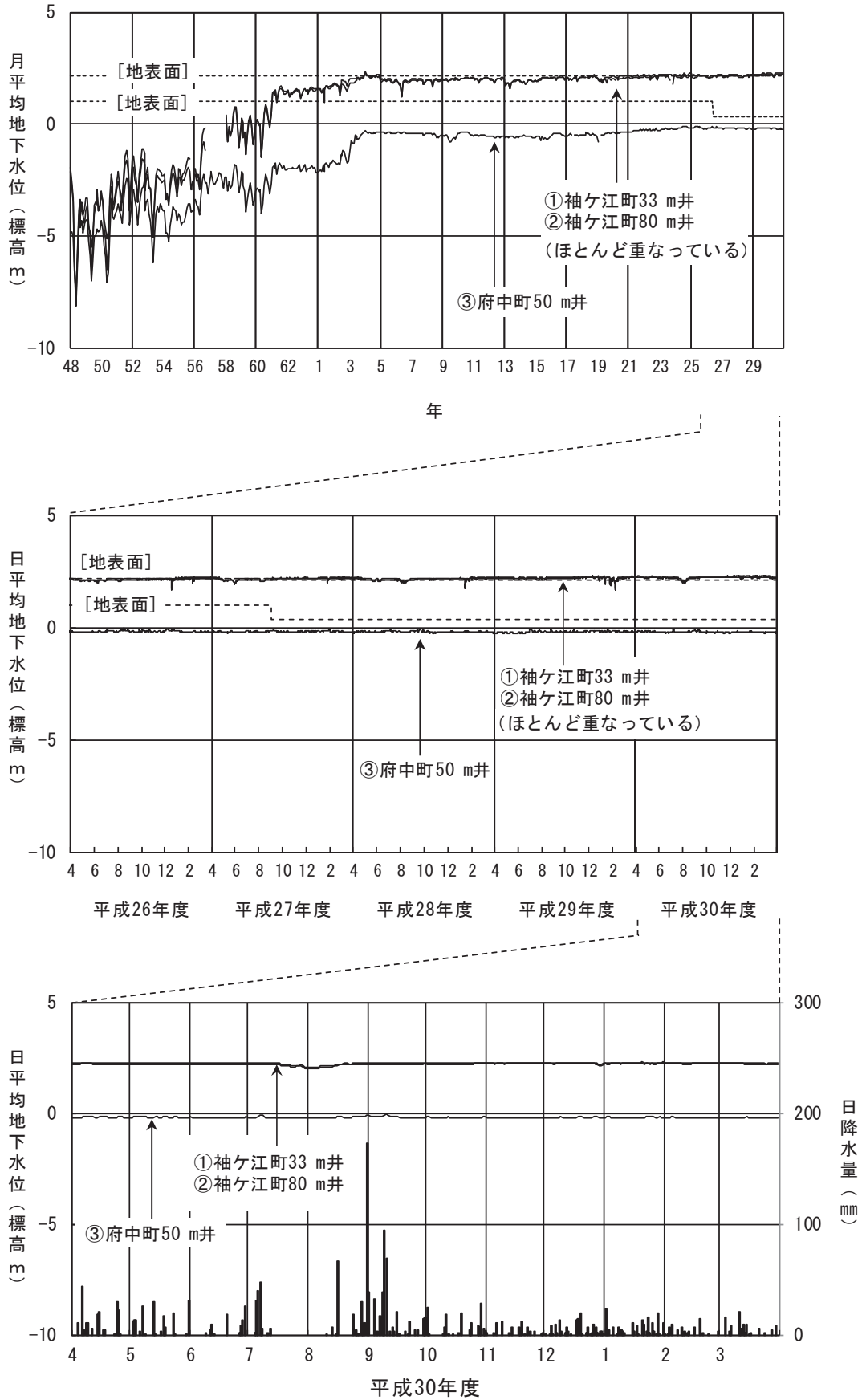
図 3-2-3 地下水位(七尾市袖ヶ江町、府中町)
