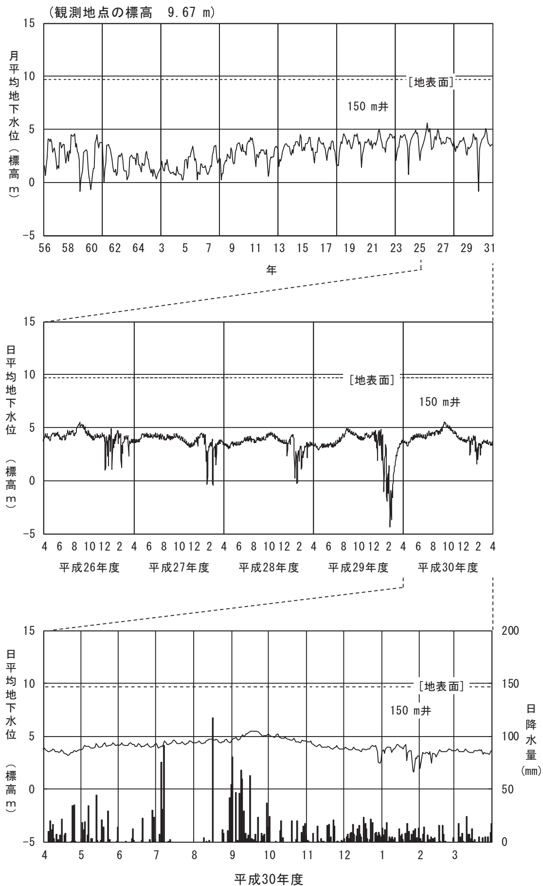
図 2-2-3(9) 地下水位 (⑨金沢市新保本)
