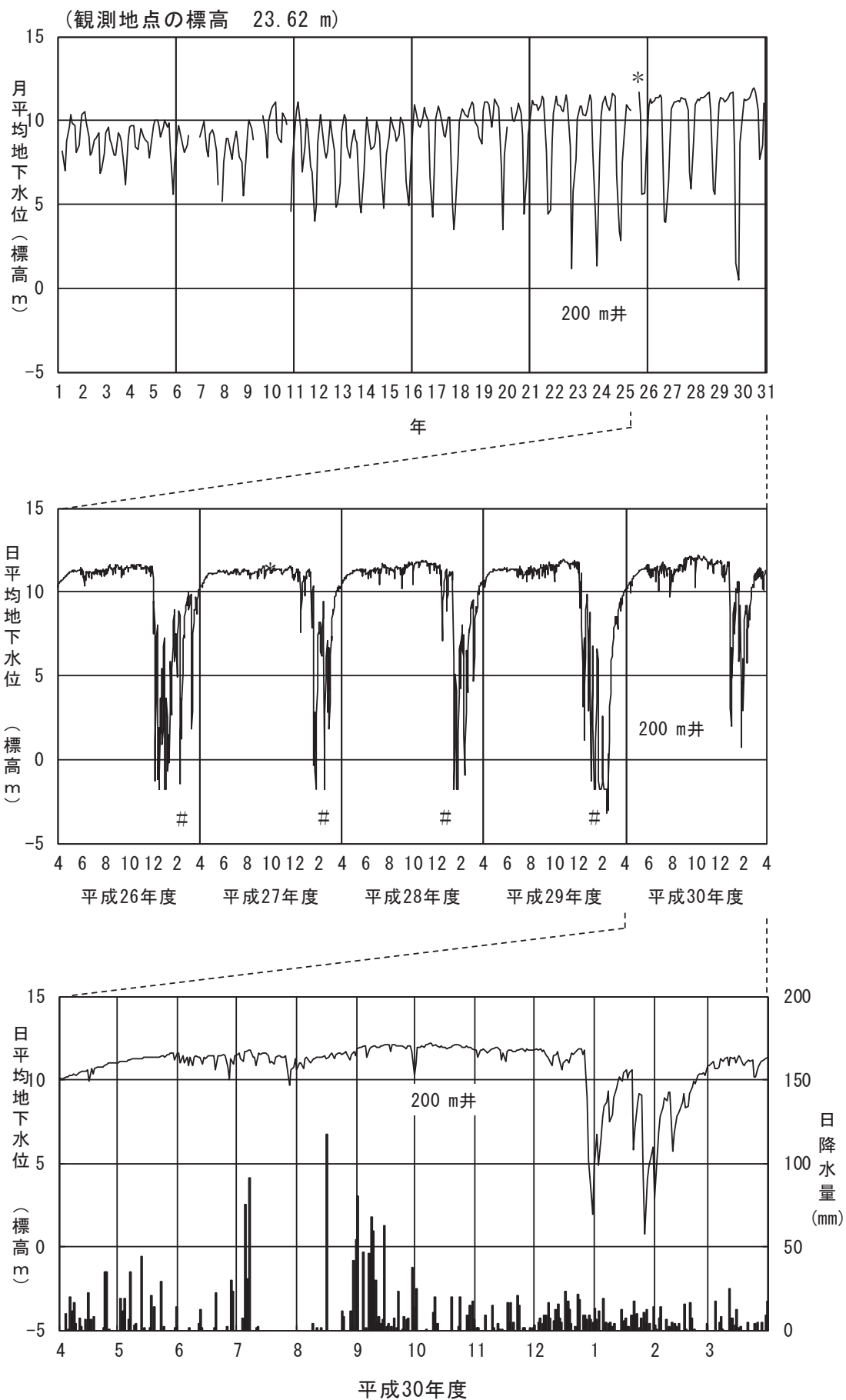
図 2-2-3(7) 地下水位 (⑦金沢市大手町)
