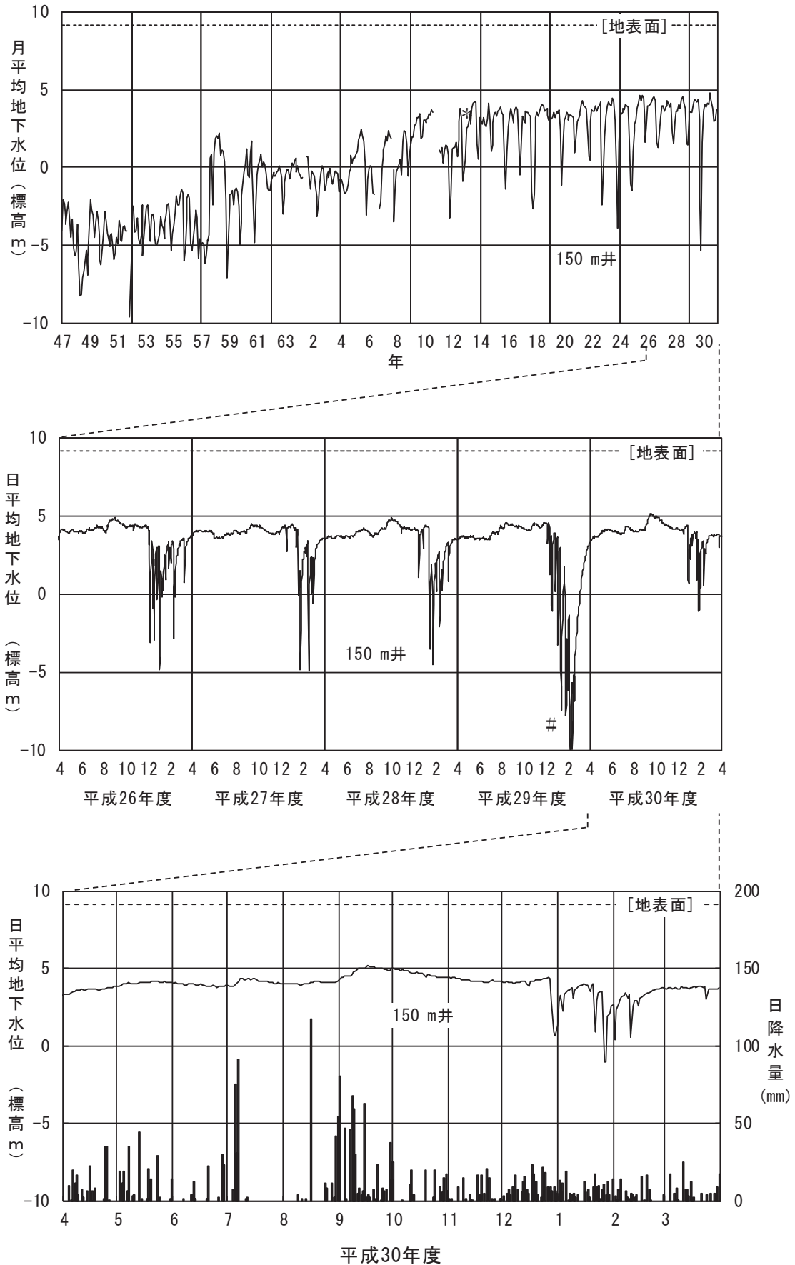
図 2-2-3(6) 地下水位 (⑥金沢市昭和町)
