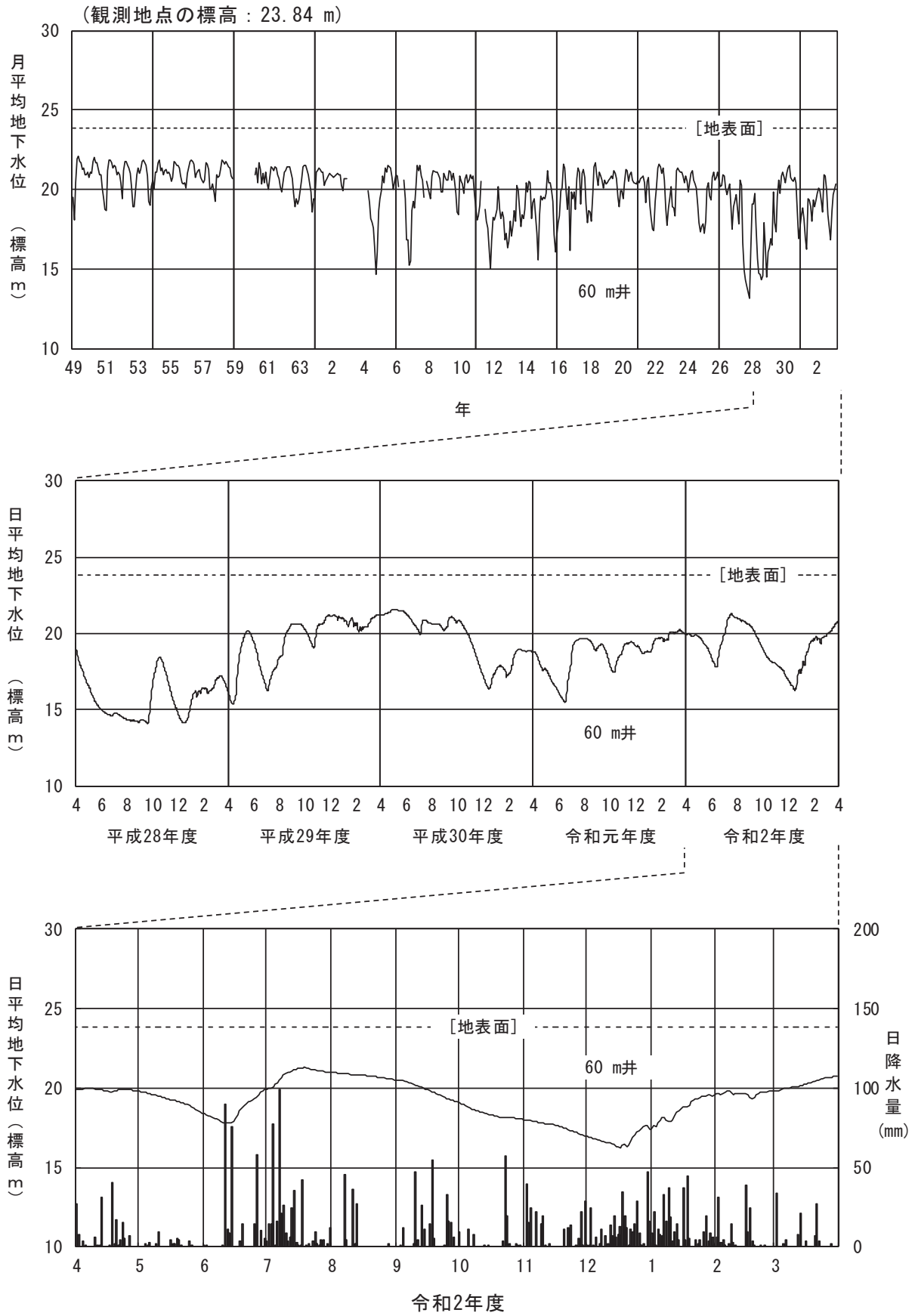
図 2-2-3 (22) 地下水水位 (㊸能美市北市)
