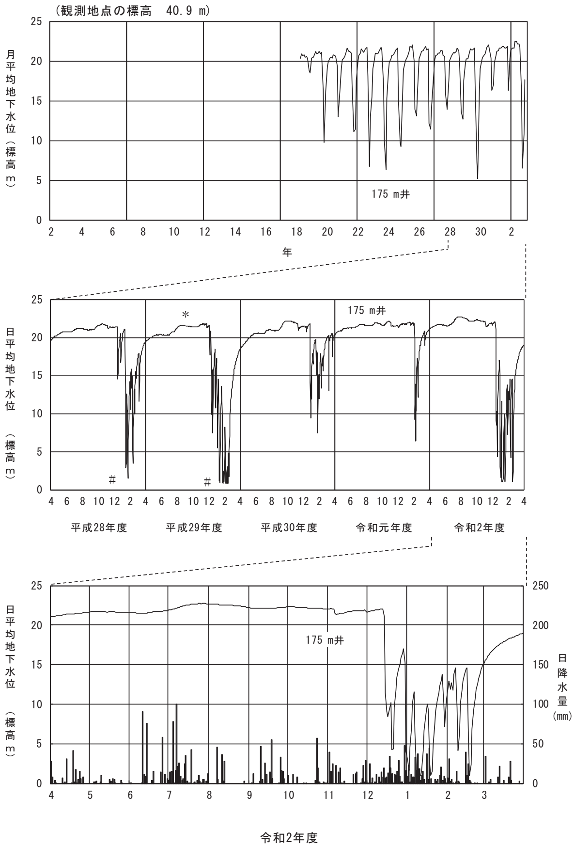
図 2-2-3(10) 地下水水位 (⑩金沢市泉野出町)
