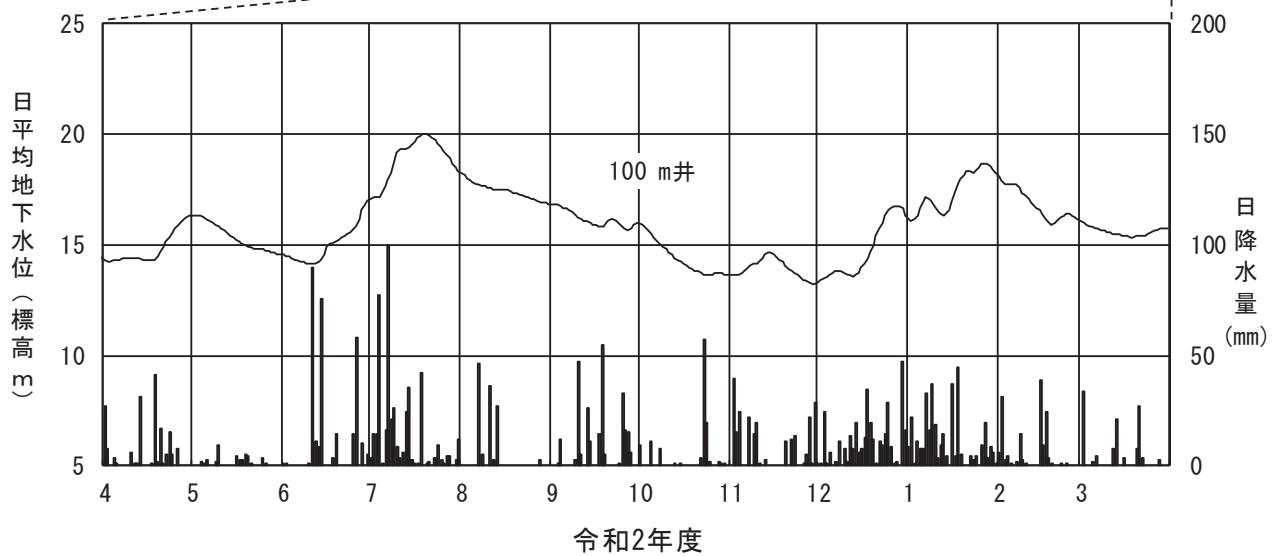
図 2-2-3(20) 地下水位 (㊸白山市安吉町)
