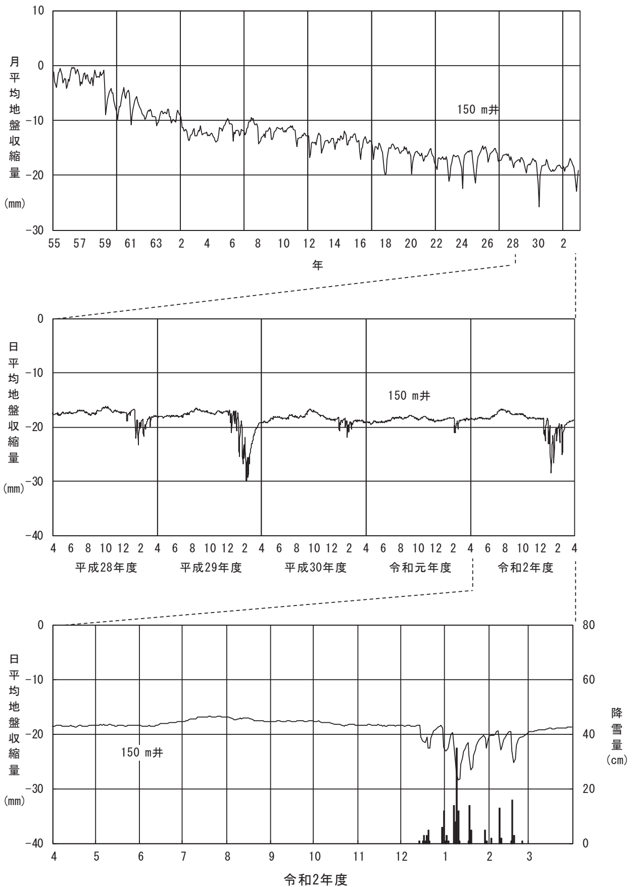
図 2-2-2 (4) 地盤収縮量 (④金沢市東力町)
