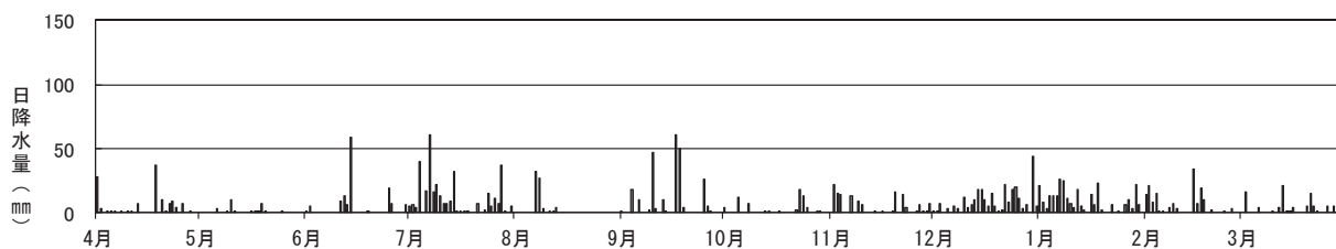
図 3-2-5 七尾地域気象観測所の日降水量(令和2年度)
