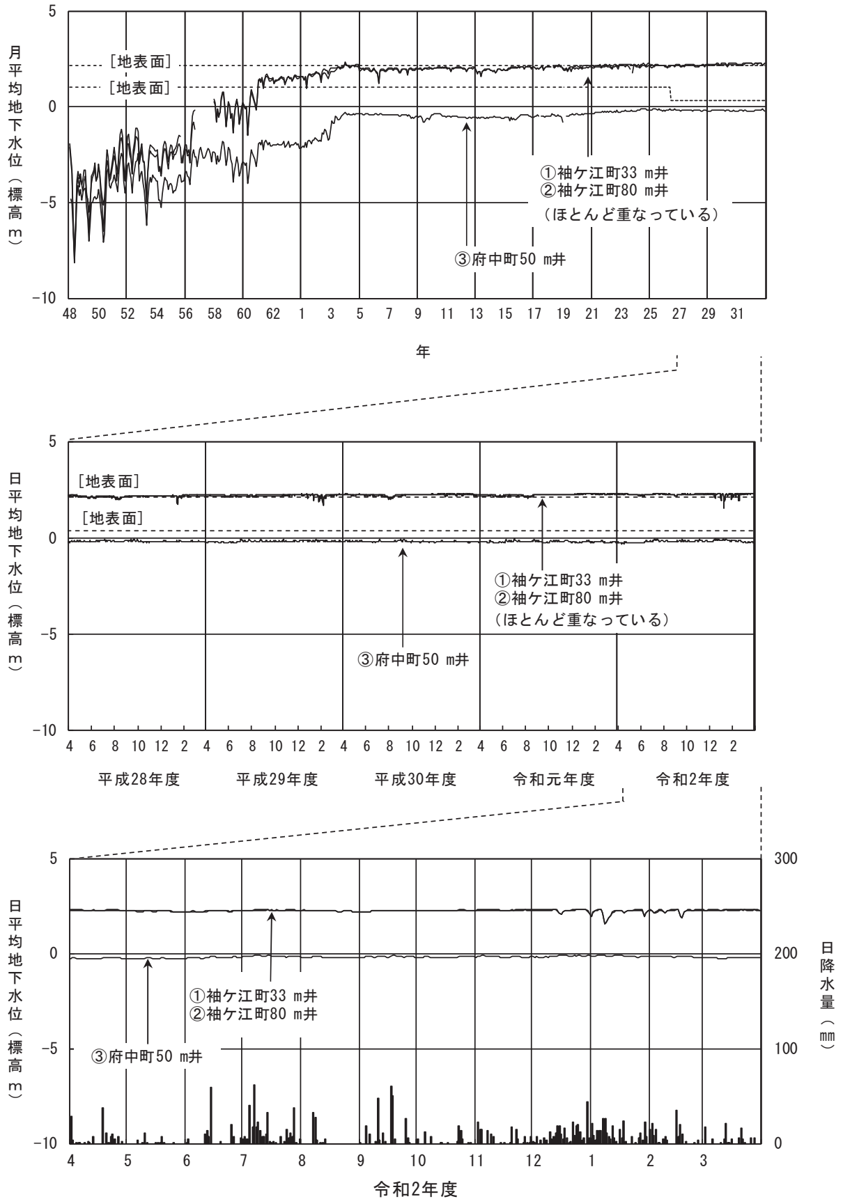
図 3-2-3 地下水水位(七尾市袖ヶ江町、府中町)
