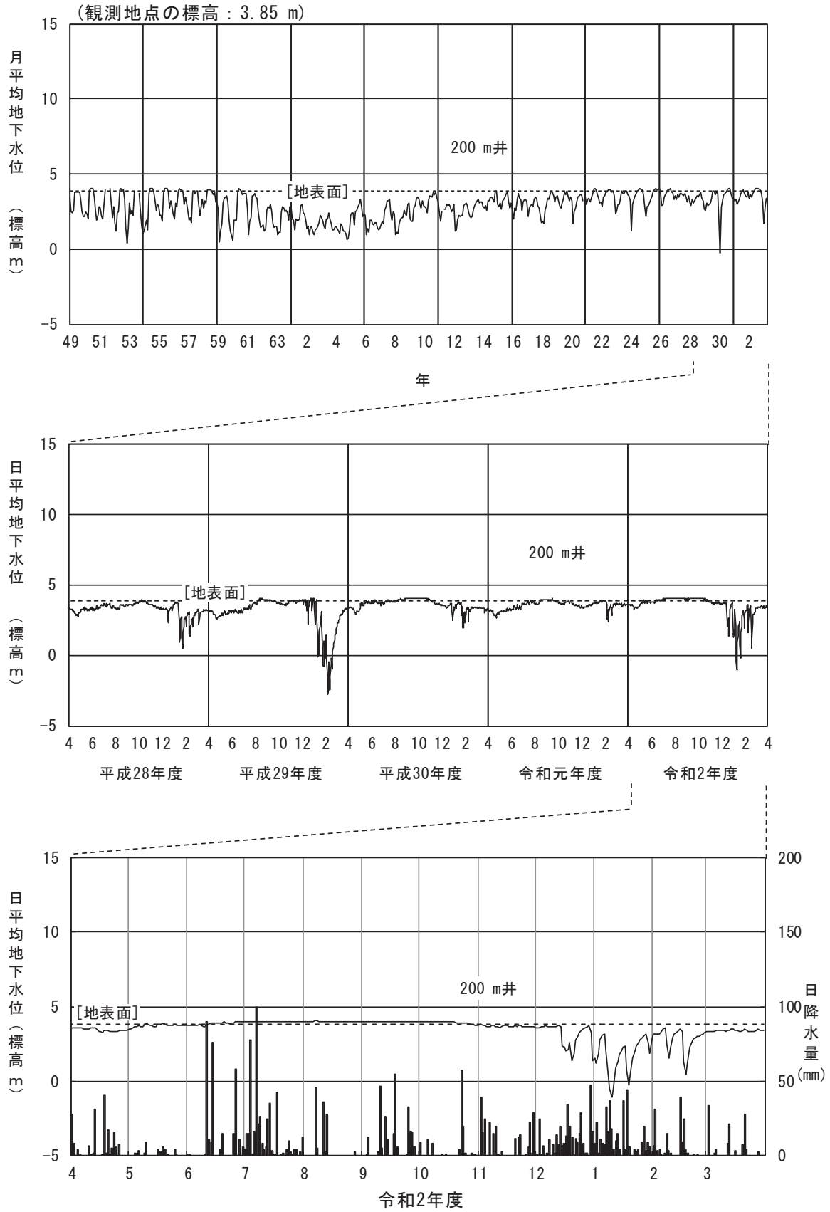
図 2-2-3 (15) 地下水位 (⑮金沢市福増町)
