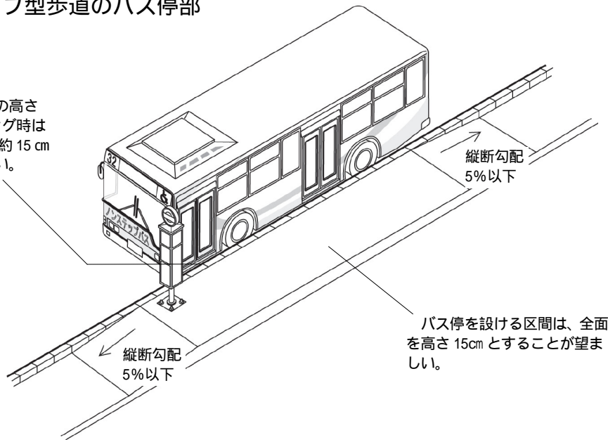
図 2-7 マウントアップ型歩道のバス停部
