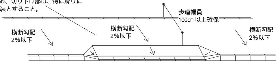
図 2-7 マウントアップ型歩道のバス停部
