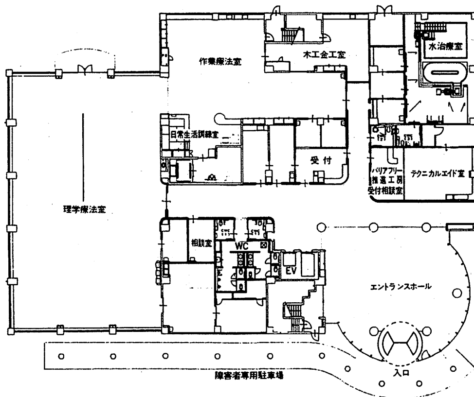
【1階平面図】
