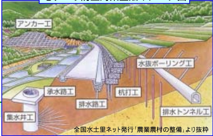
地すべり防止対策工法イメージ図
