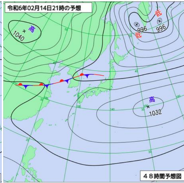
14日21時予想天気図
