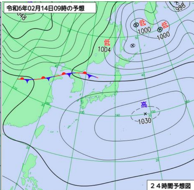
14日9時予想天気図
