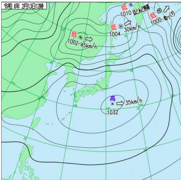
13日12時実況天気図
