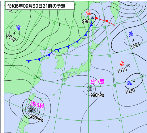
30日 21時 予想天気図
