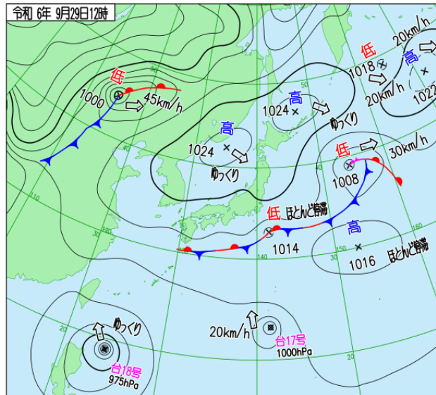
29日 12時 実況天気図
