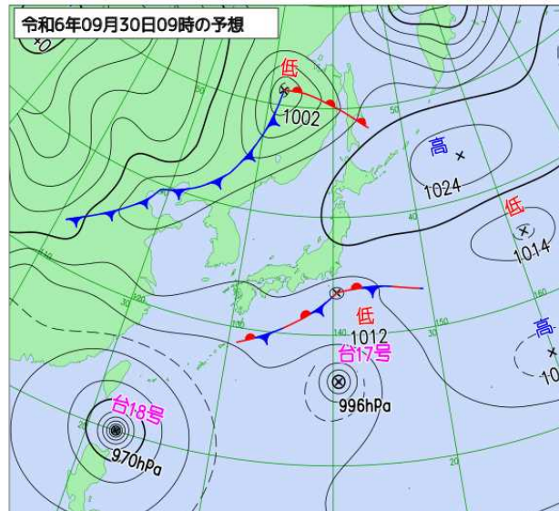
30日 9時 予想天気図
